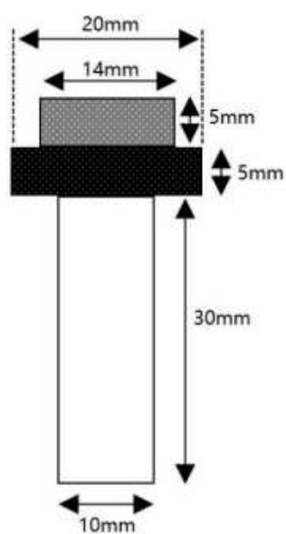
图 4.1-8 双砂轮规格尺寸图（灰色区域 1#粒径磨料、黑色区域镀 2#粒径磨料）
