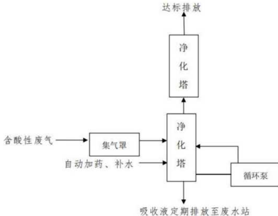
图 8.3-2 工艺流程简图
