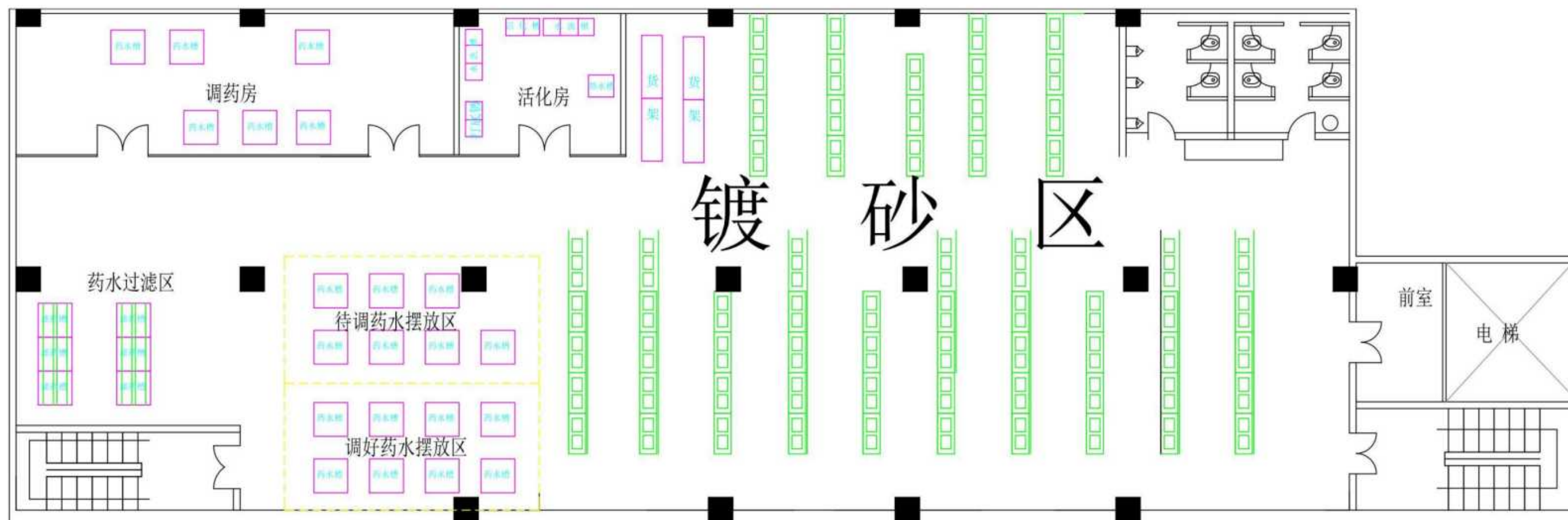
图 4.1-16 能源动力楼 8 楼车间平面布局图（砂轮生产线）
