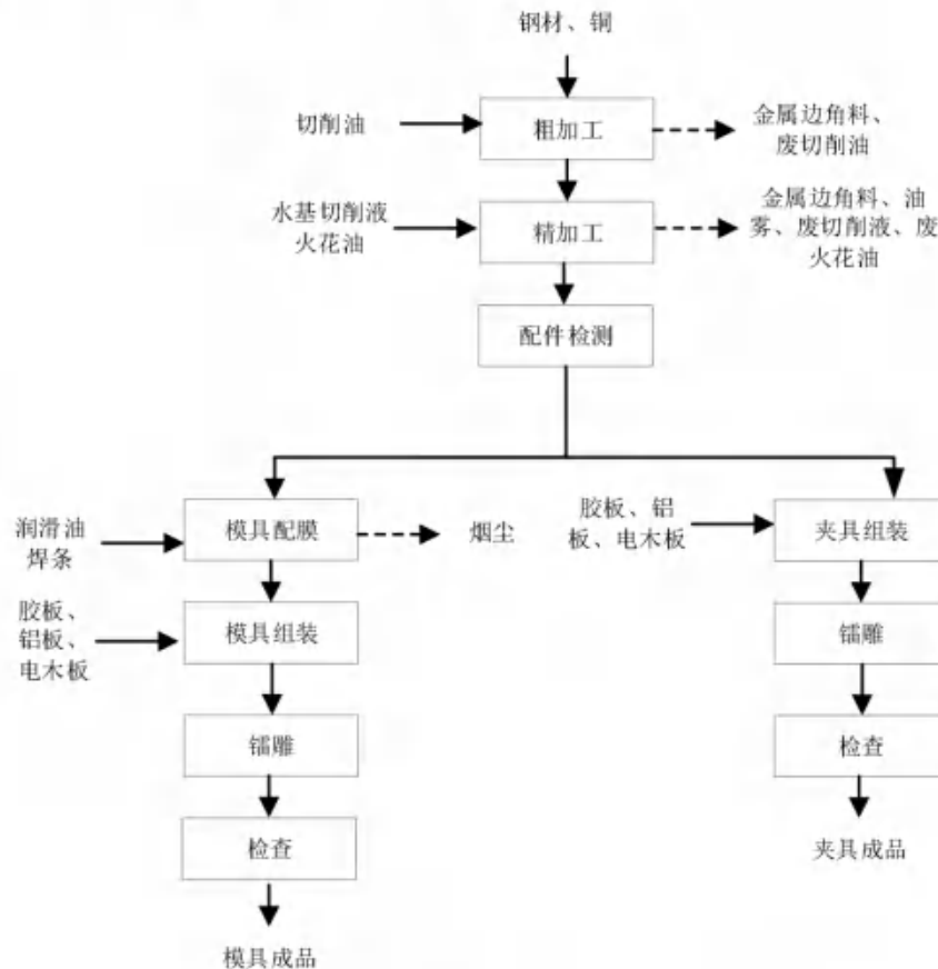
图 3.3-10 五金模&塑胶模&夹具生产工艺流程图
