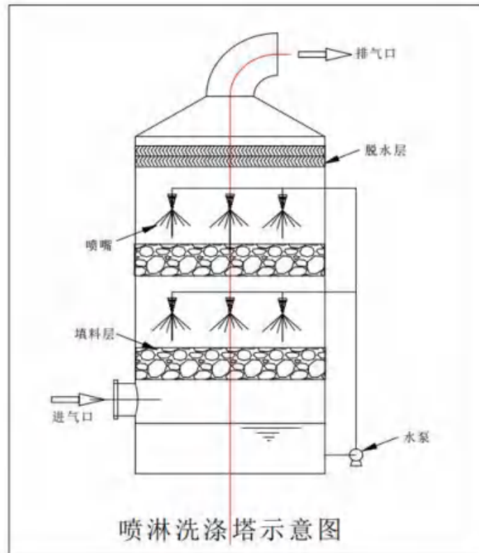
图 8.3-3 喷淋净化塔结构图
