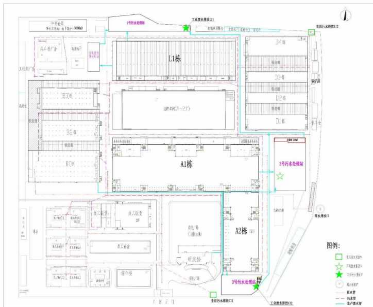
图 9.6-3 工业废水、车间废水、雨水、生活污水管网图
