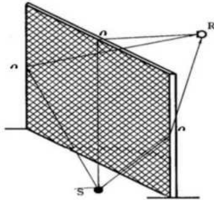
图 1.1-1 在有限长声屏障上不同的传播途径
