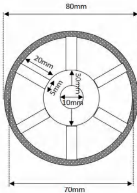
图 4.1-9 Φ80mm 大砂轮规格尺寸图
