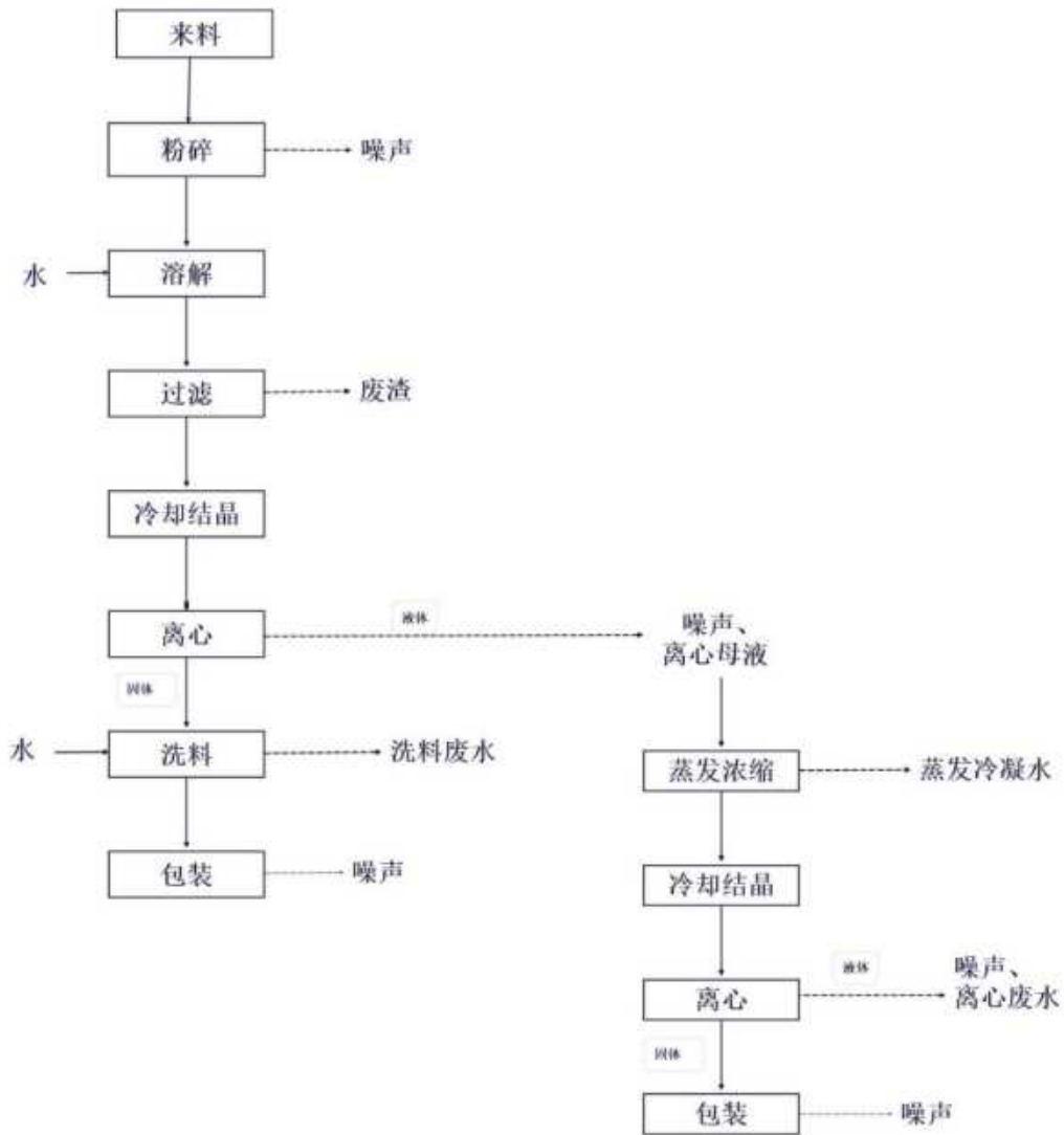
图 3.3-18 硝酸钾回收利用生产流程图
