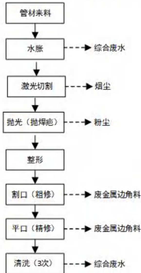
图 4.2-8 保温杯外壳、内胆、外壳底片、内胆底片生产工艺流程图
