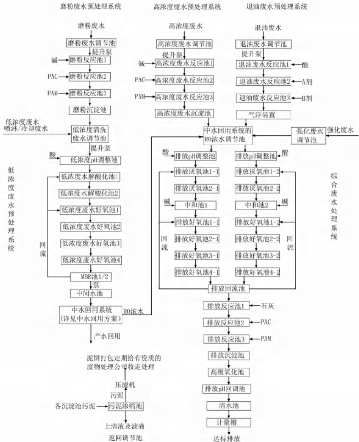
图 3.4-1 现有项目废水处理工艺流程图 (t/d)
