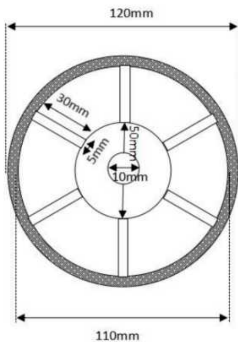
图 4.1-10 \Phi 120\text{mm} 大砂轮规格尺寸图
