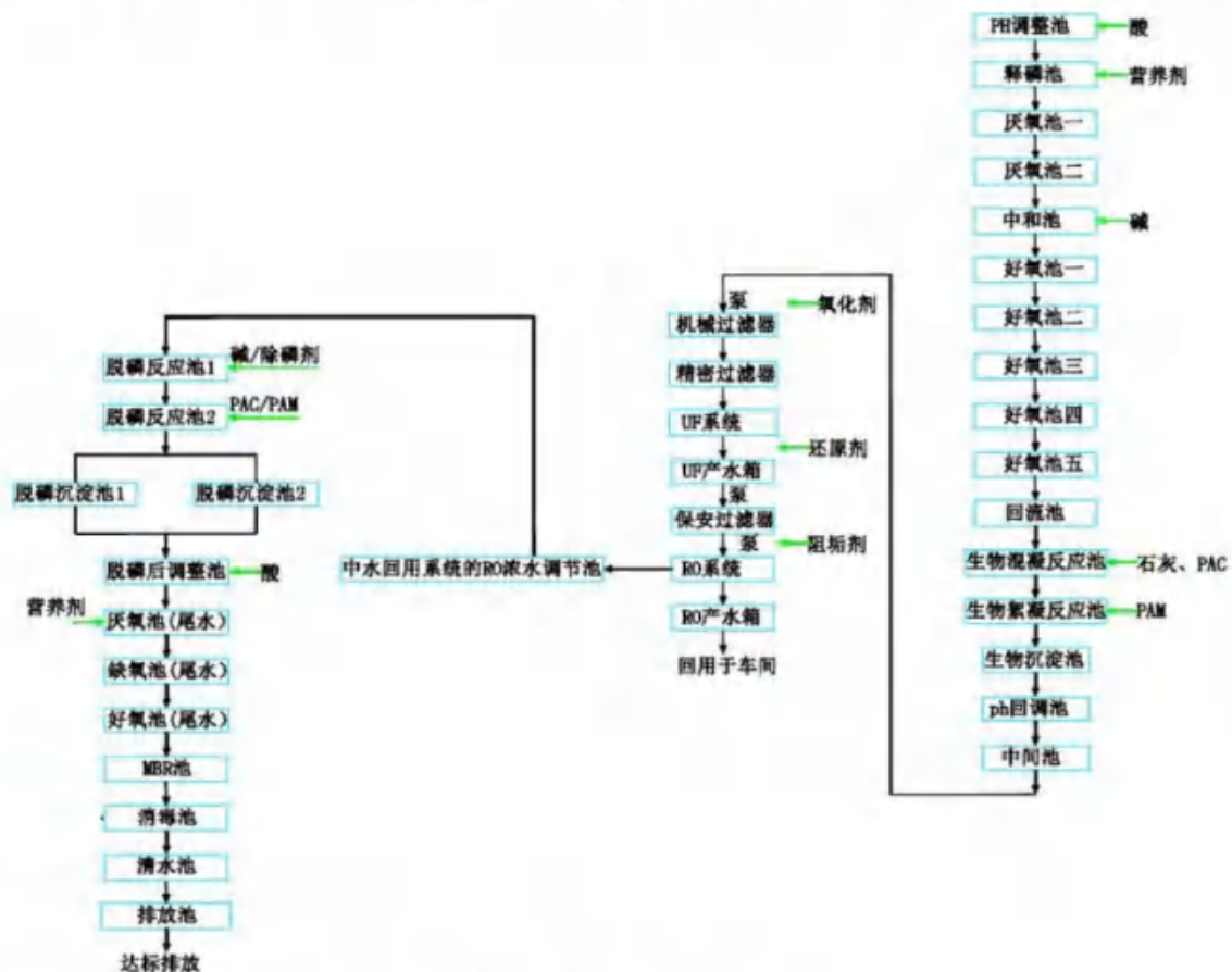
图 7.1-2 1 号废水处理站工艺流程图
