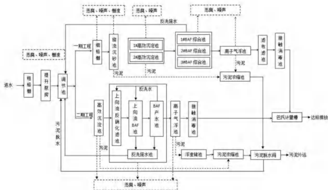
图 7.1-1 惠阳经济开发区污水处理厂处理工艺流程图
