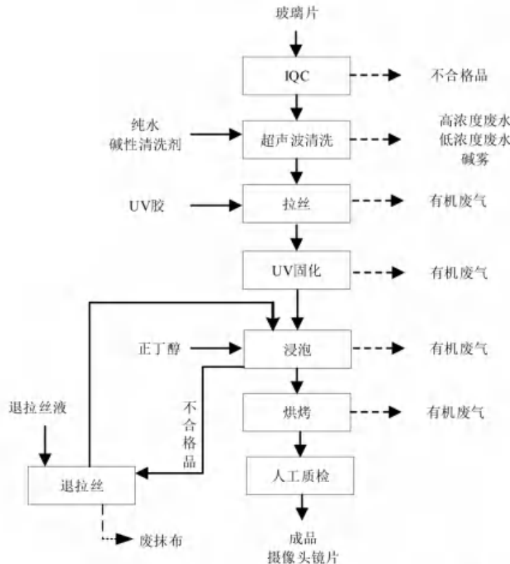
图 3.3-15 摄像头镜片生产工序
