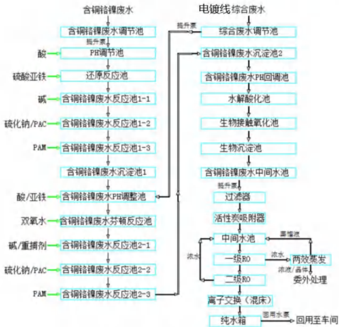
图 8.2-1 新建的 4 号废水处理站处理工艺流程
