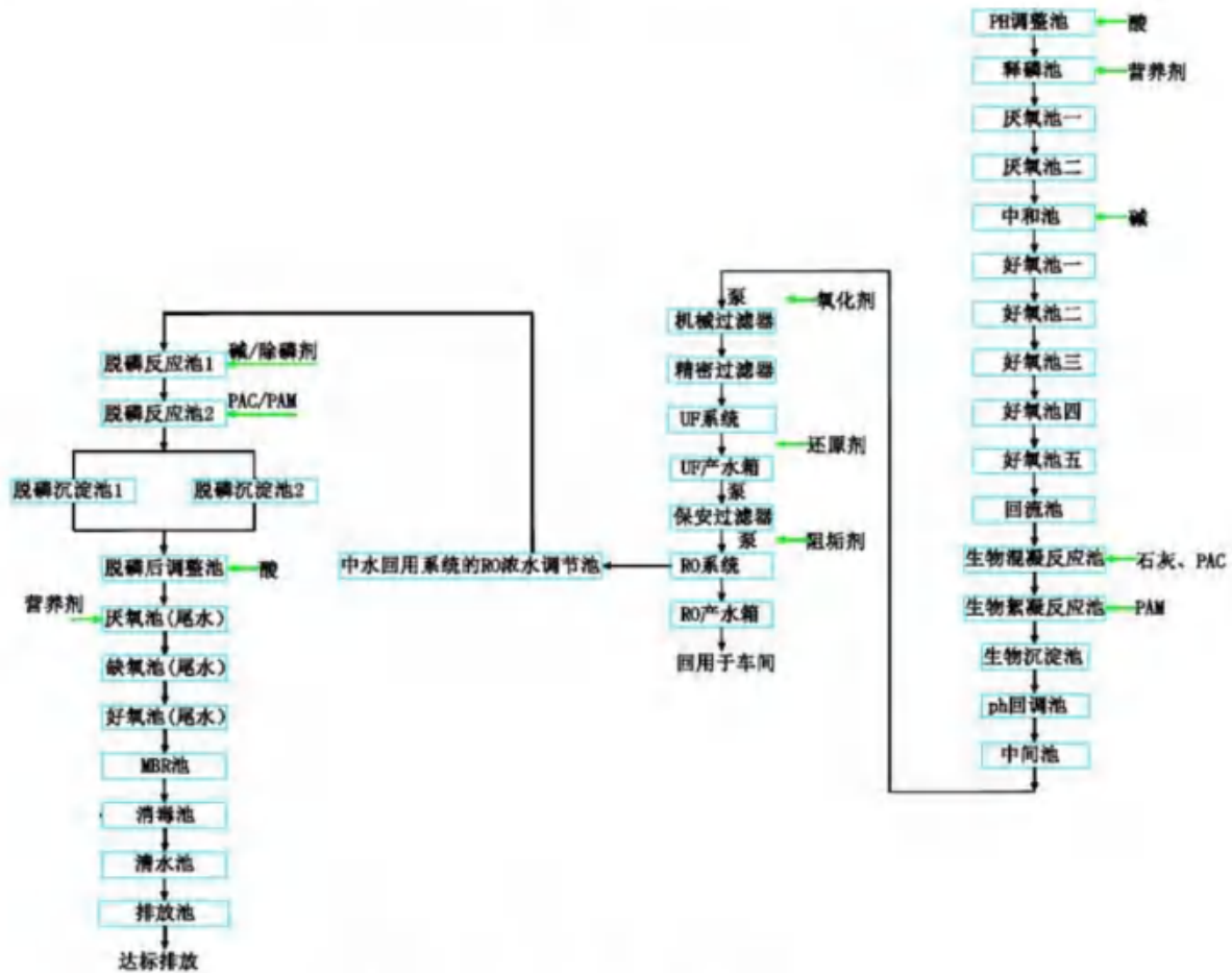
图 4.4-2 1号废水处理站工艺流程图
