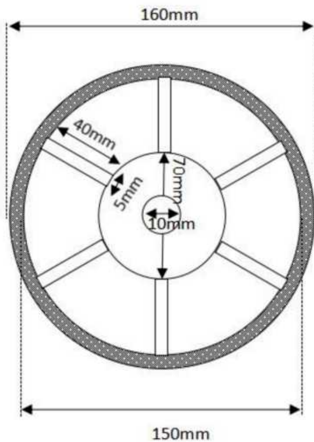
图 4.1-11 \Phi 160\text{mm} 大砂轮规格尺寸图
