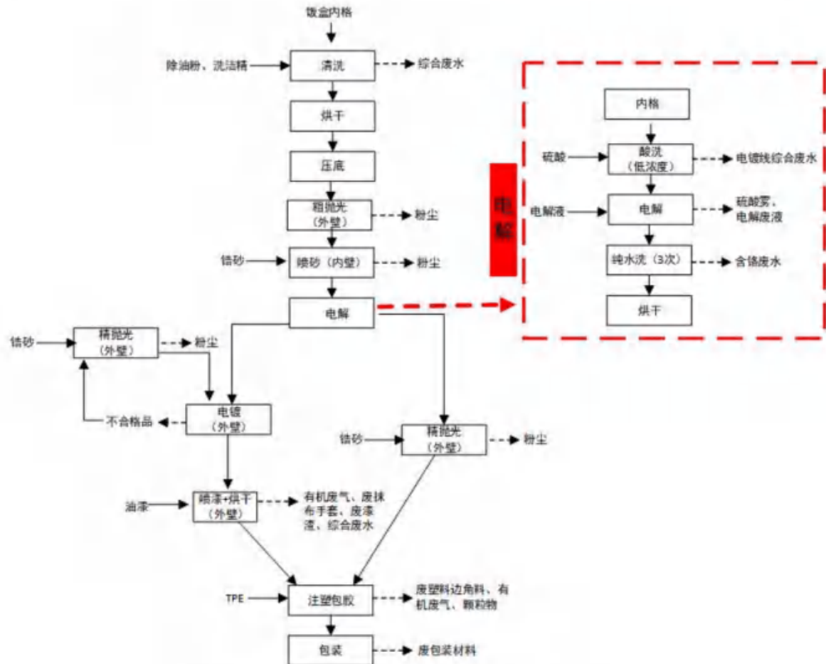
图 4.2-4 保温饭盒内格表面处理工艺流程图
