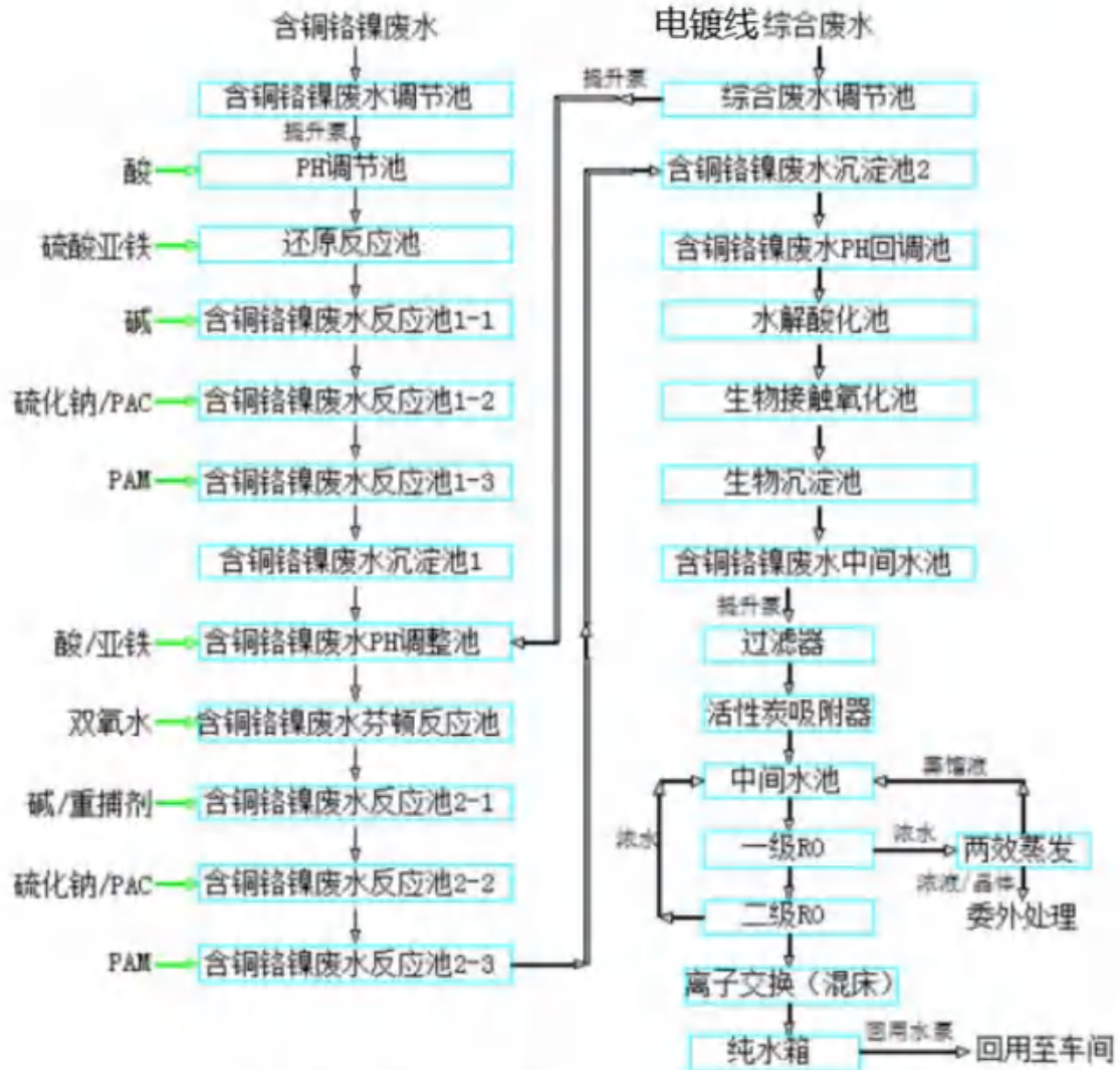
图 4.4-1 4 号废水处理站工艺流程图
