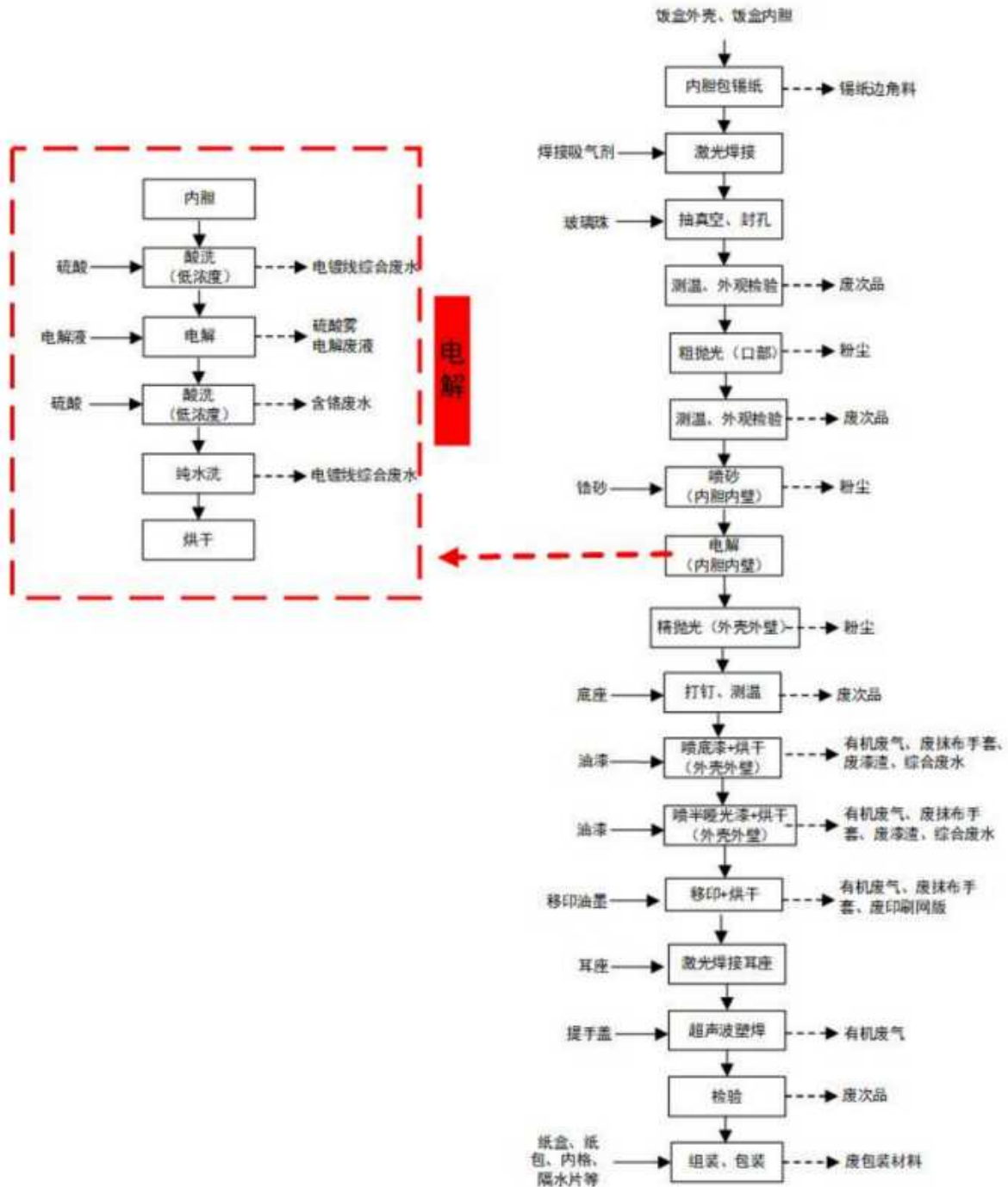
图 4.2-1 保温饭盒主体生产工艺流程图
