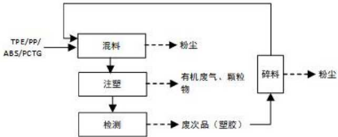
图 4.2-9 保温杯杯盖、底座生产工艺流程图
