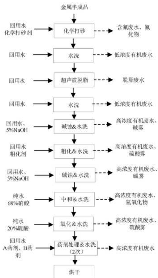
图 3.3-2 T 处理工艺流程及产污环节图
