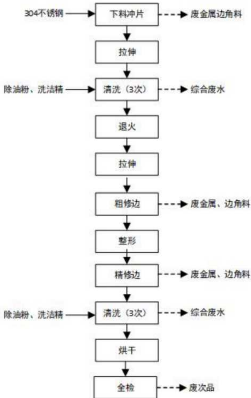
图 4.2-2 保温饭盒内胆、外壳、内格生产工艺流程
