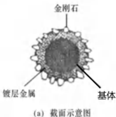
图 4.1-3 金刚石砂轮工作区域结构示意图
