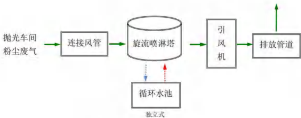
图 8.3-1 工艺流程简图
