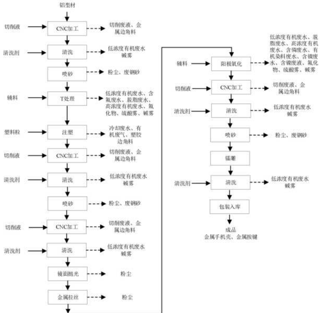
图 3.3-1 金属加工项目生产工艺流程及产污环节图
