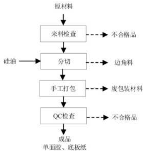
图 3.3-17 单面胶、底板纸生产流程图
