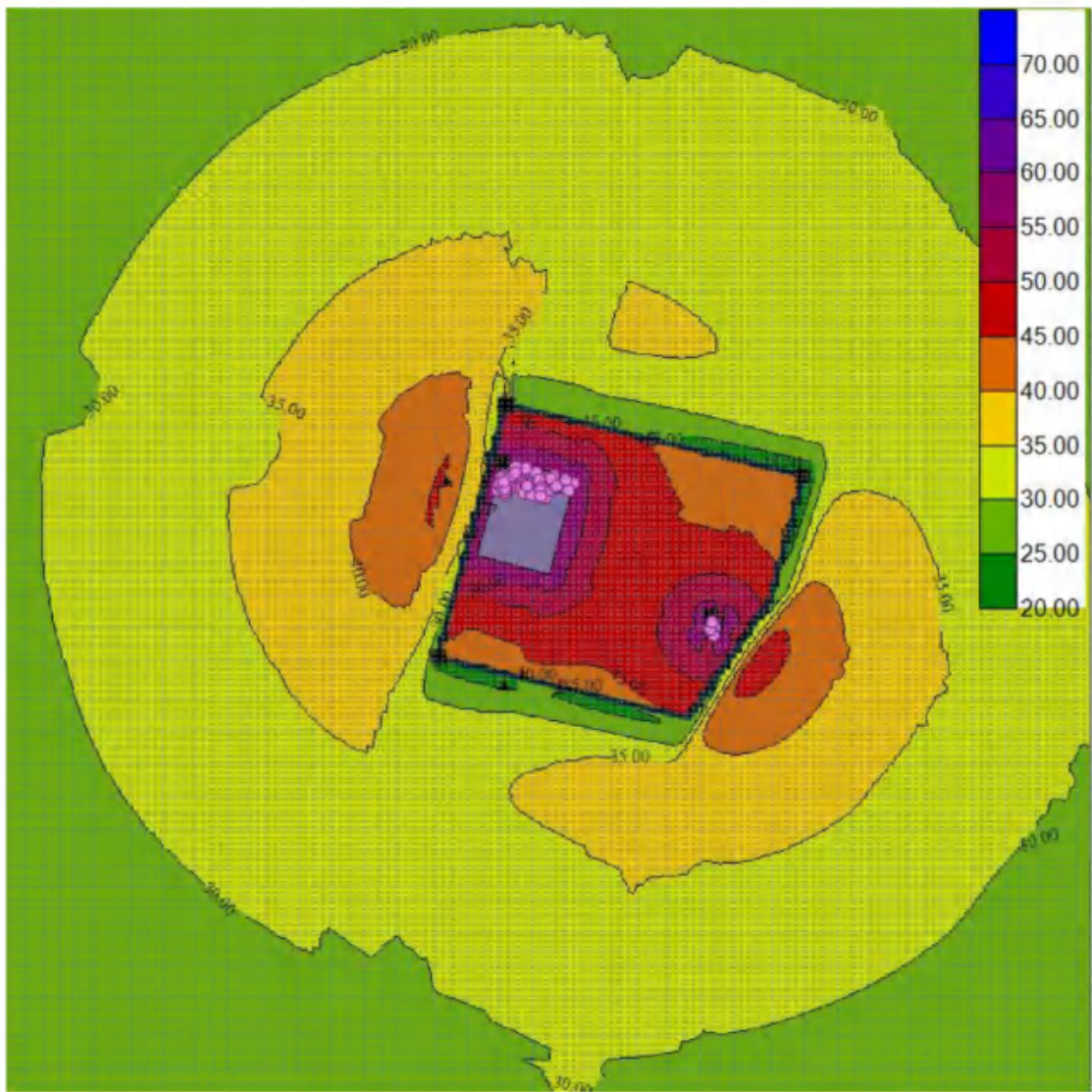
图 7.3-1 噪声贡献值等声级线图
