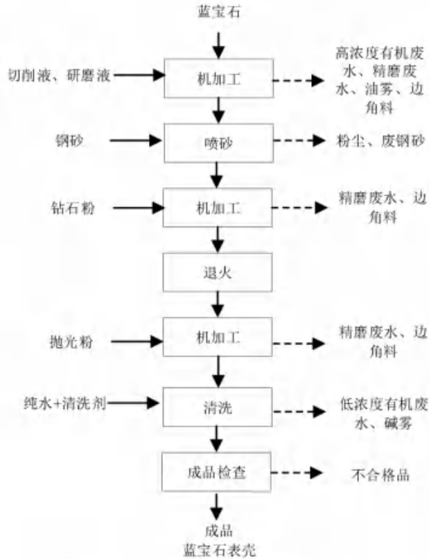
图 3.3-9 蓝宝石表壳的主要生产工艺及产污节点图
