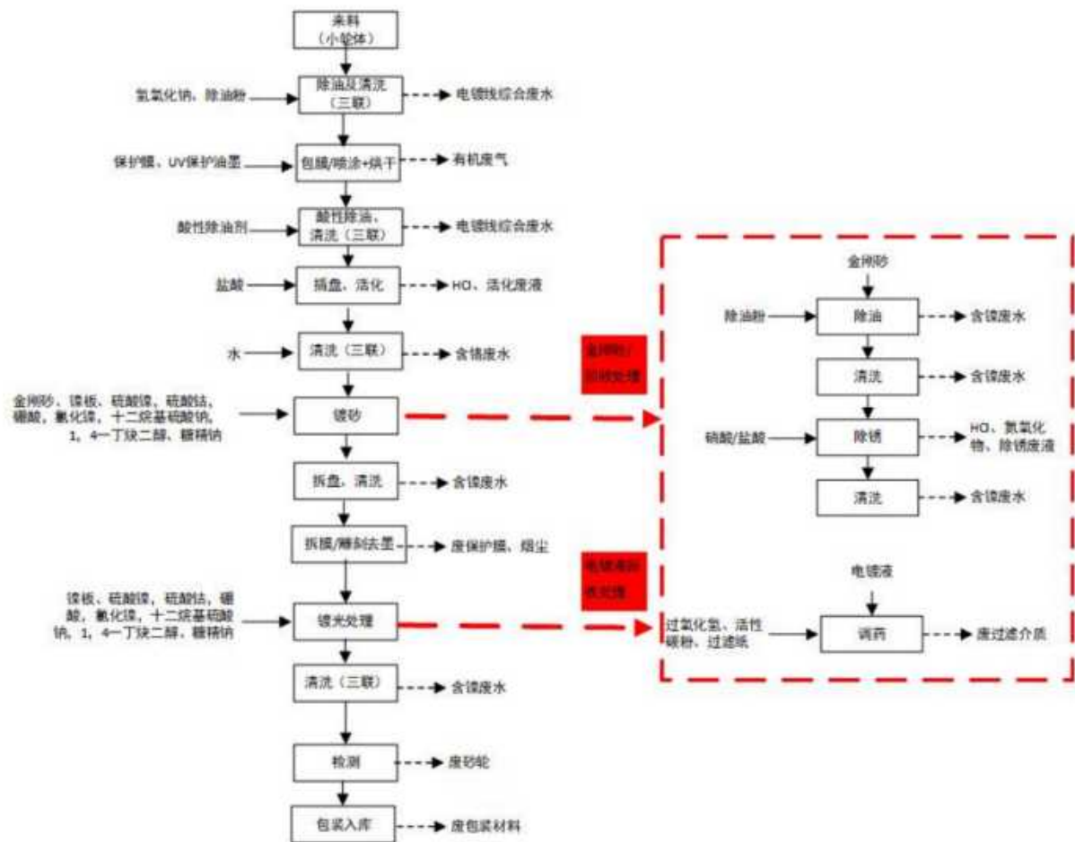
图 4.2-11 小砂轮生产工艺流程图
