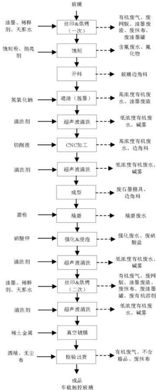
图 3.3-4 车载触控玻璃项目生产工艺流程及产污环节图
