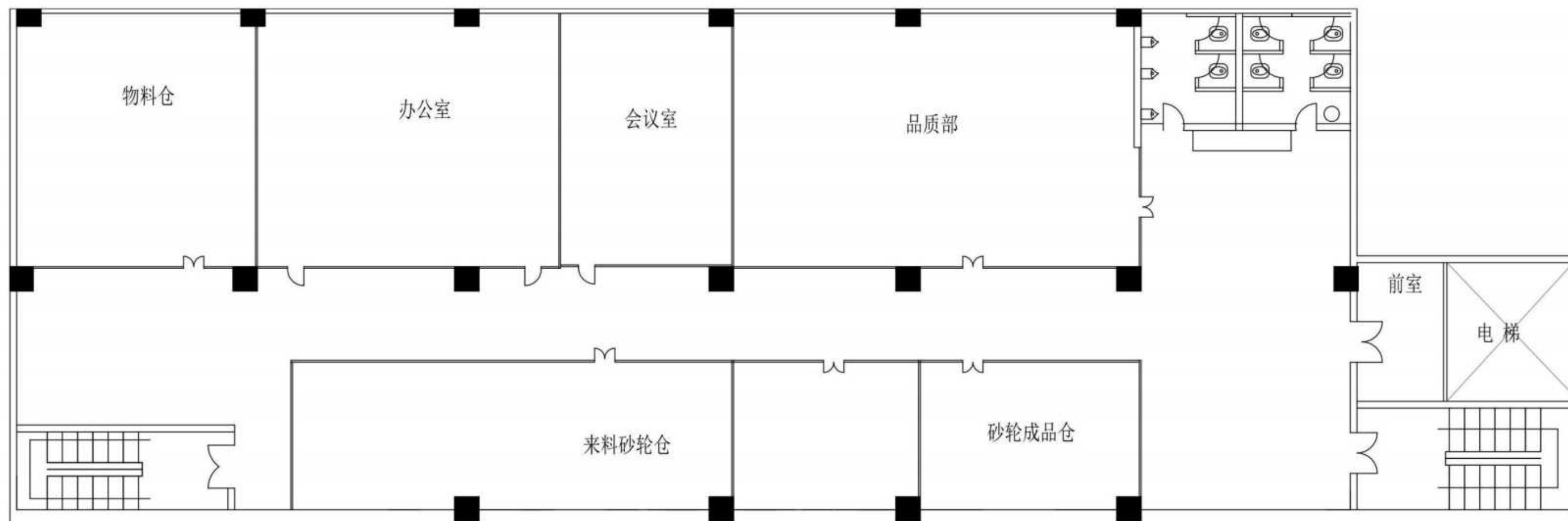
图 4.1-13 能源动力楼 5 楼车间平面布局图（砂轮生产线）
