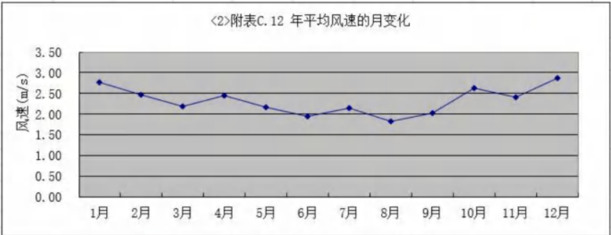
图 7.2-13 惠阳气象站年平均风速的月变化图
