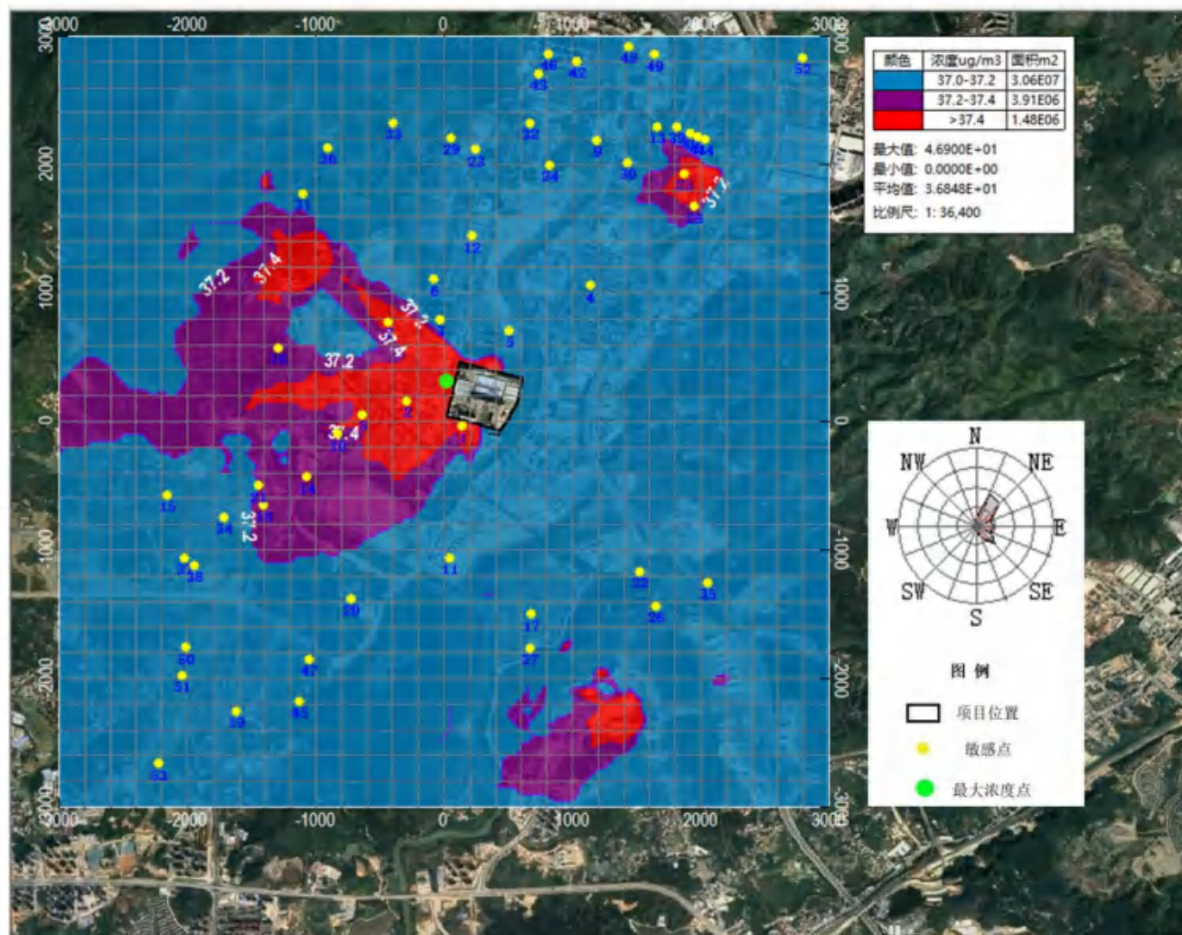
图 7.2-29 PM2.5 日平均浓度分布图
