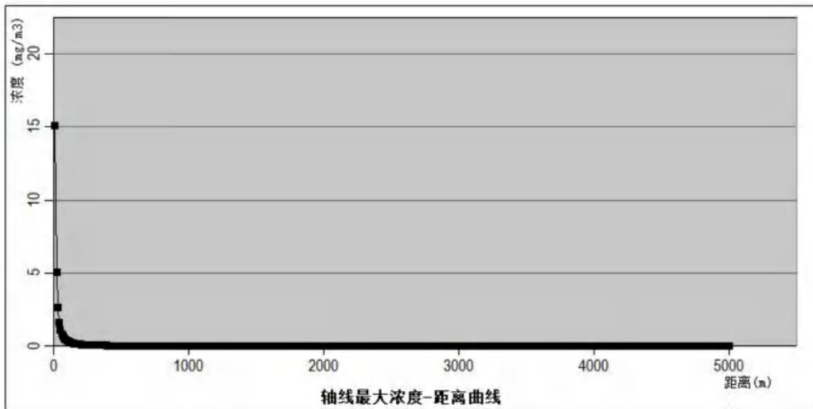
图 9.6-2 火灾伴生/次生 CO 排放在下风向不同距离处的最大浓度（最不利气象条件）
