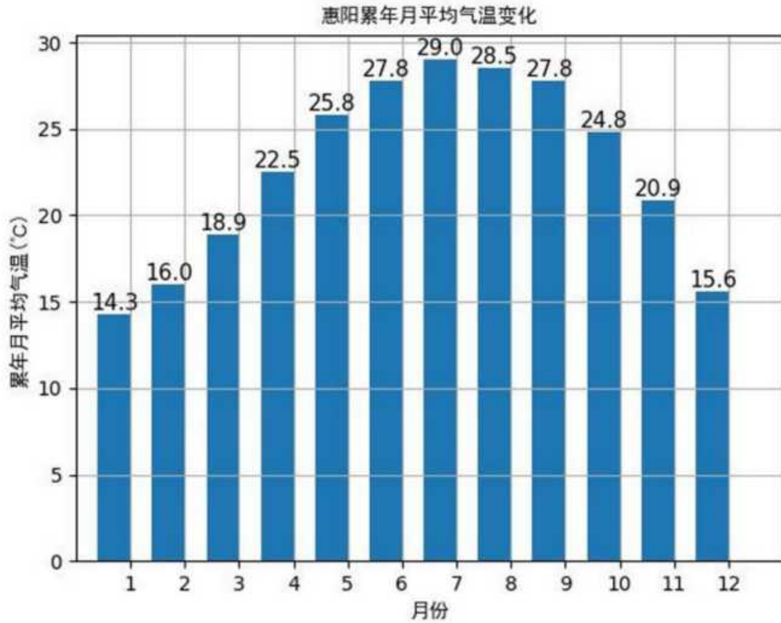
图 7.2-4 惠阳月平均气温（单位：°C）
