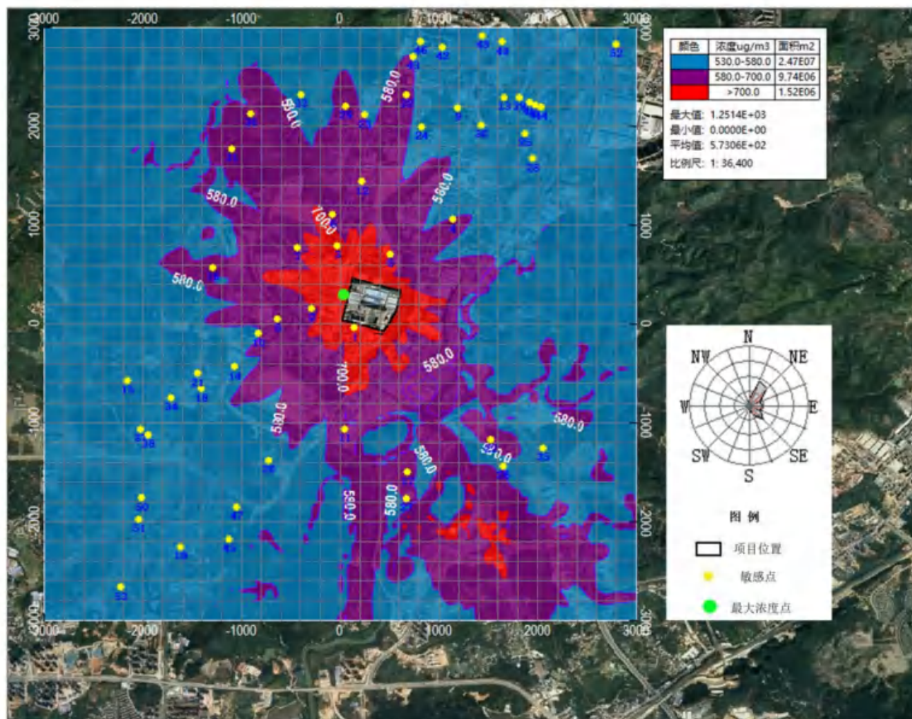
图 7.2-32 非甲烷总烃小时值平均浓度分布图
