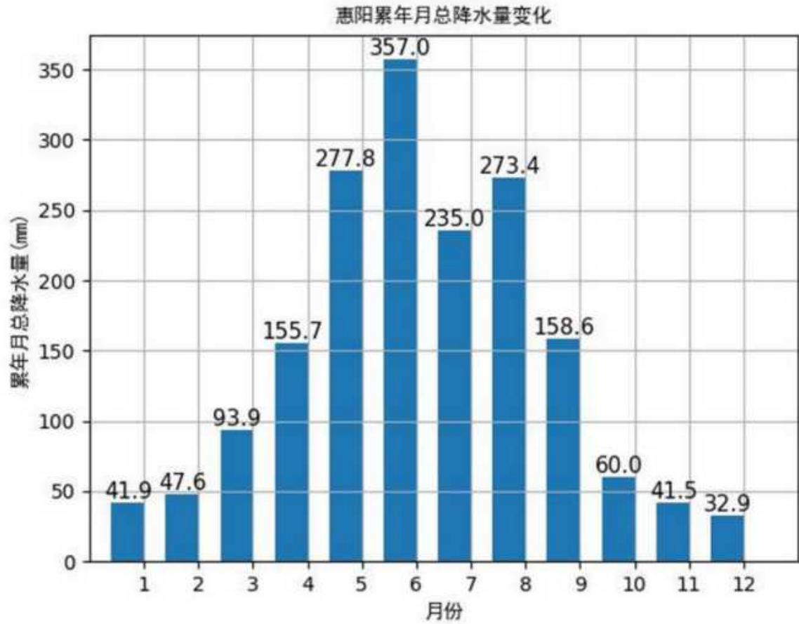
图 7.2-6 惠阳月平均降水量（单位：毫米）
