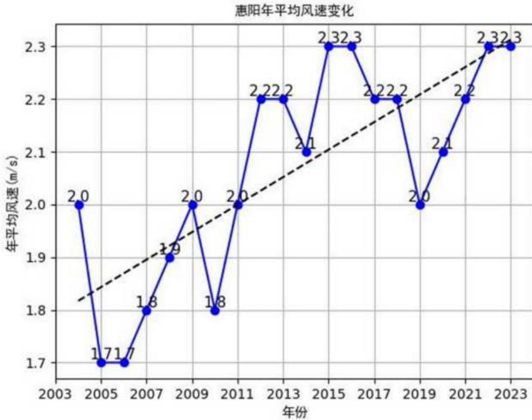
图 7.2-3 惠阳（2004-2023）年平均风速（单位：m/s，虚线为趋势线）
