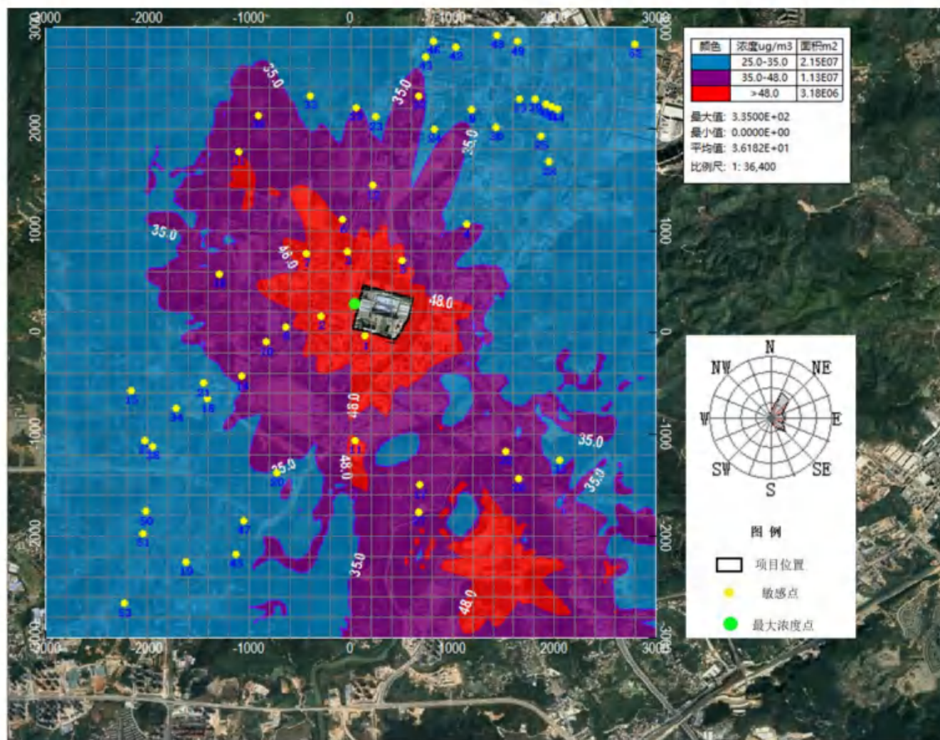
图 7.2-31 VOCs8 小时值平均浓度分布图
