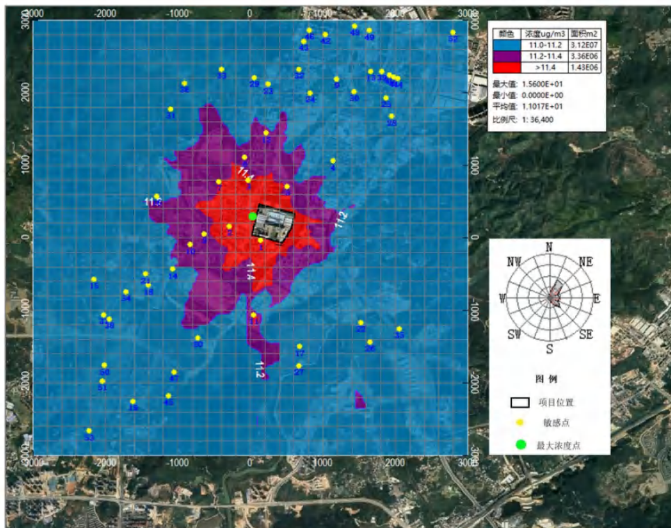
图 7.2-35 硫酸雾日平均浓度分布图
