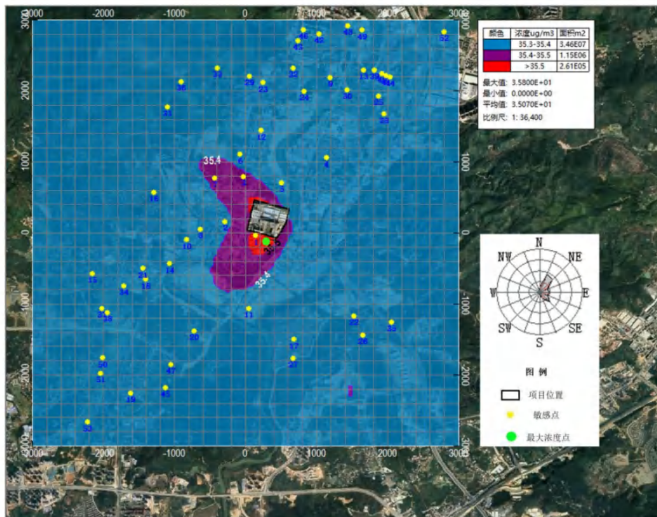
图 7.2-24 \text{NO}_x 年平均浓度分布图
