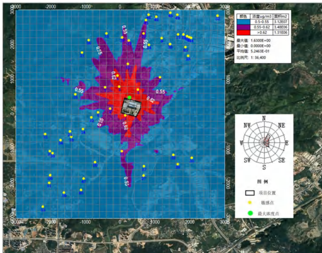
图 7.2-38 硫化氢小时值平均浓度分布图
