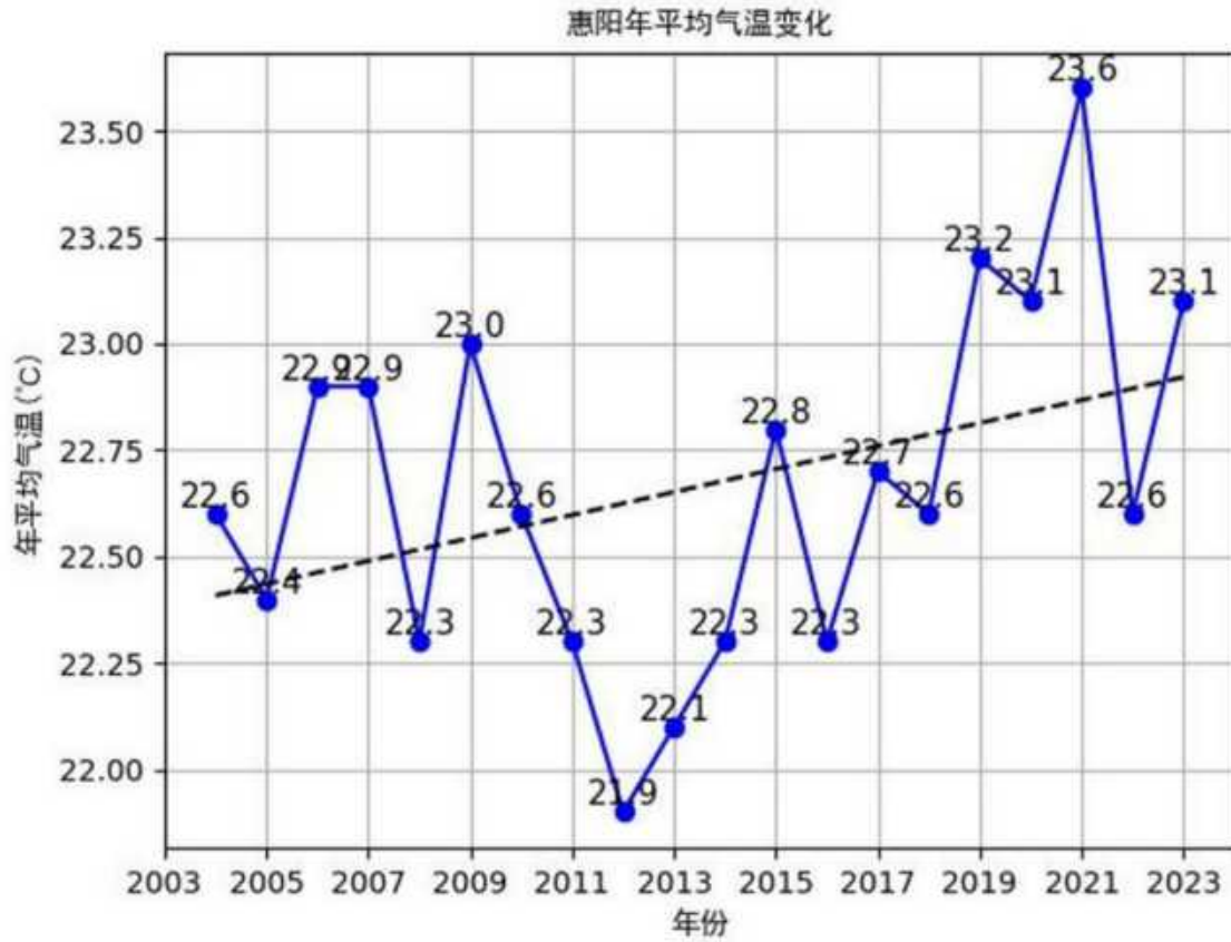
图 7.2-5 惠阳（2004-2023）年平均气温（单位：°C，虚线为趋势线）
