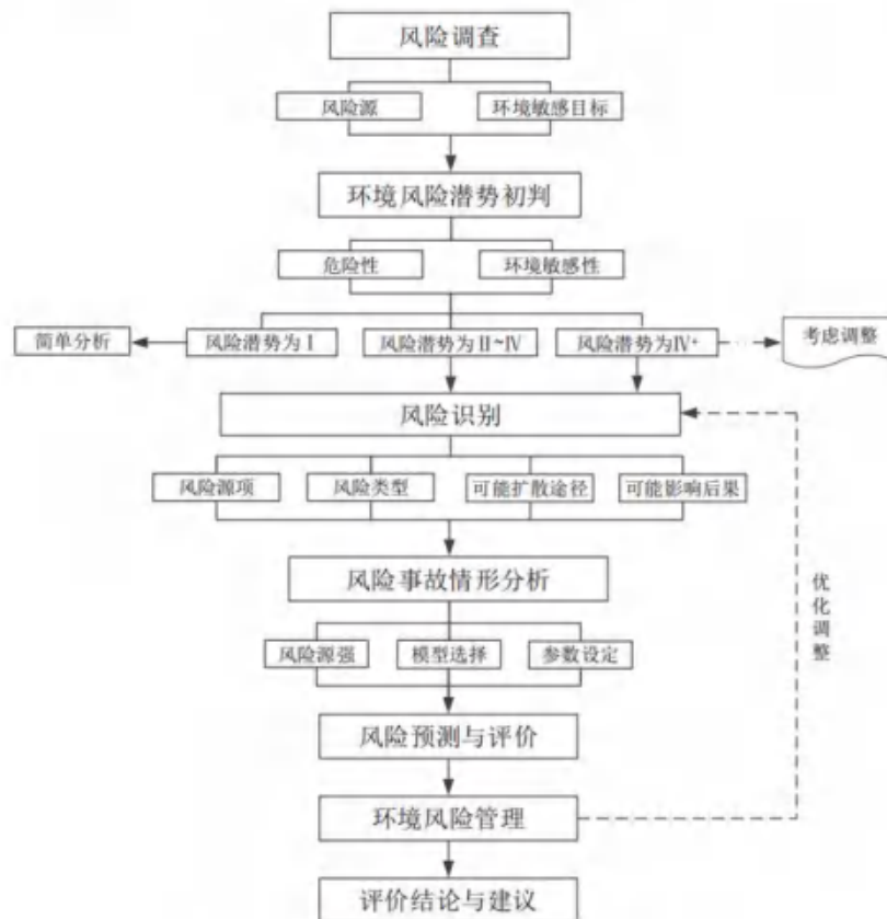
图 9.1-1 环境风险评价工作程序图
