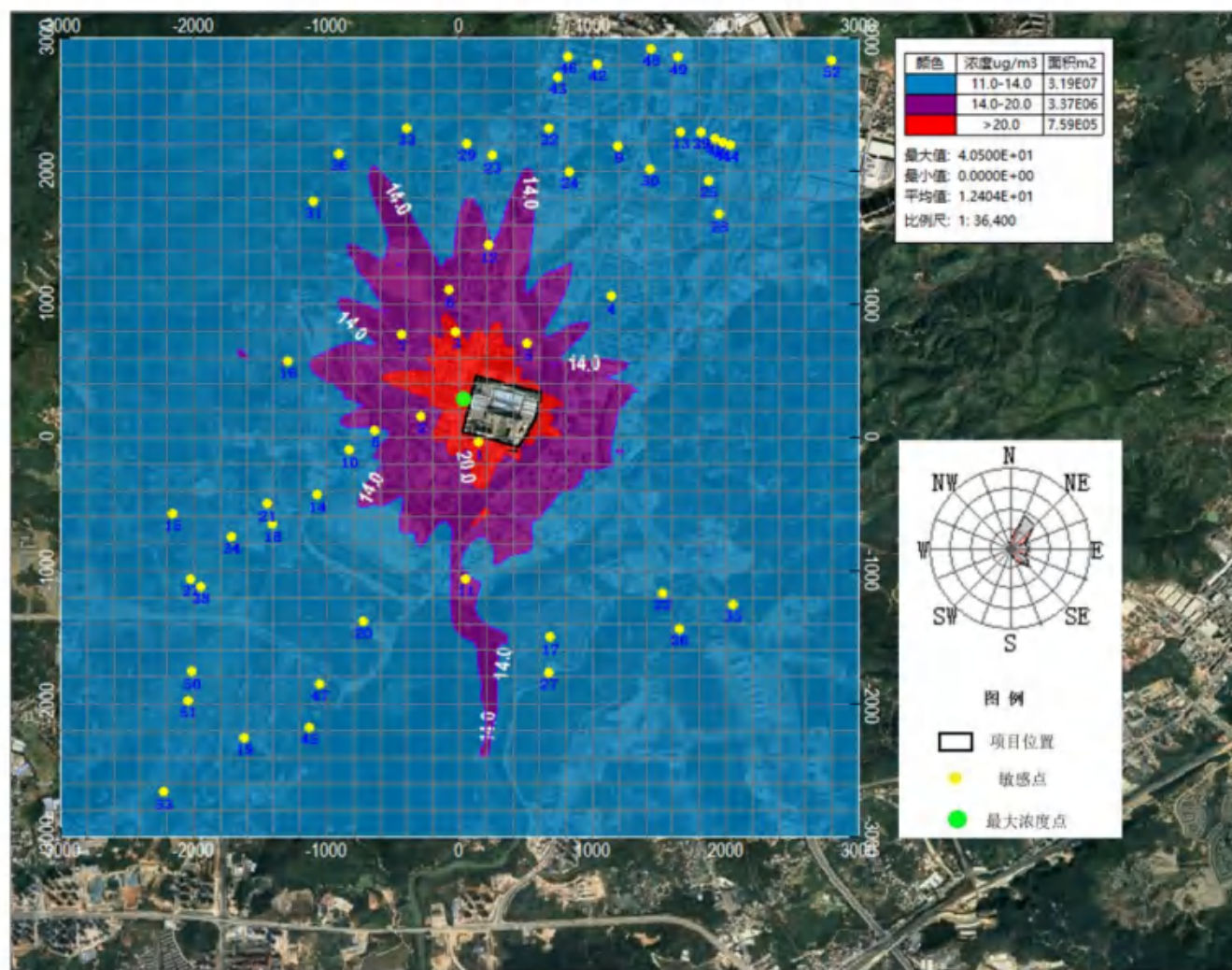
图 7.2-34 硫酸雾小时值平均浓度分布图
