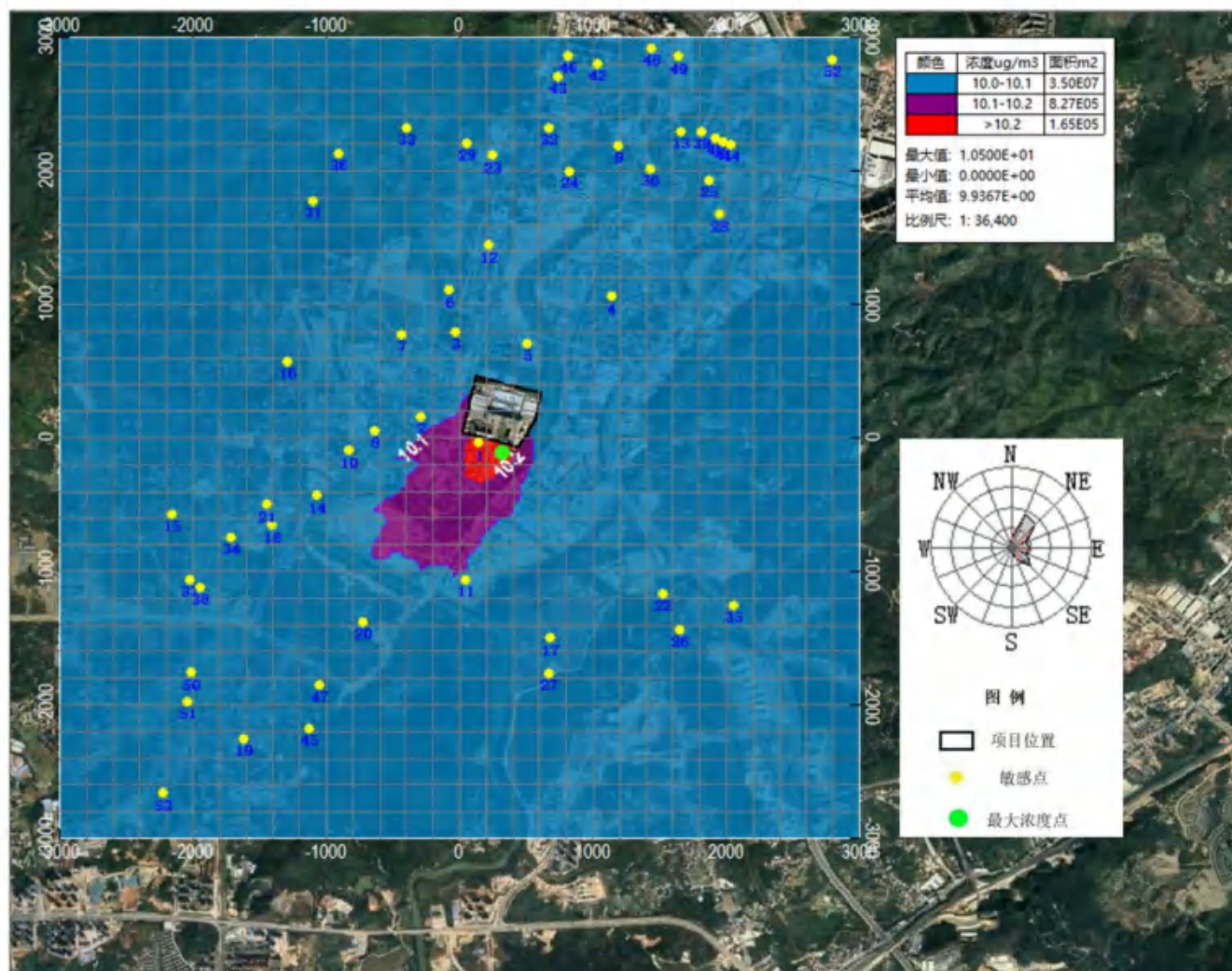
图 7.2-18 SO 2 日平均浓度分布图
