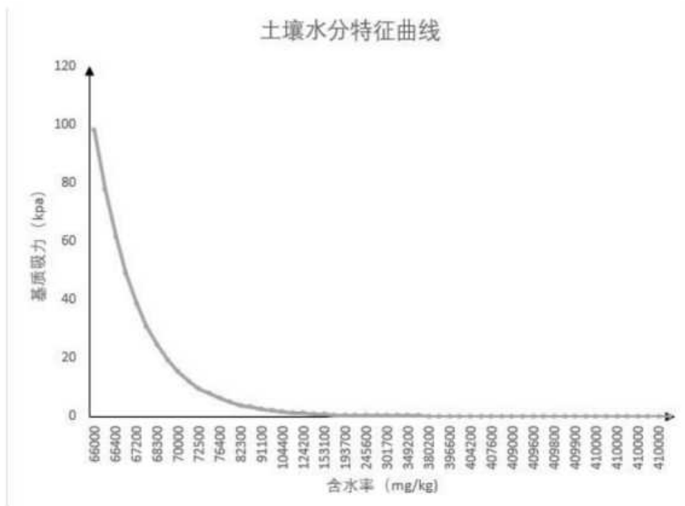
图 7.6-1 土壤水分特征曲线类型
