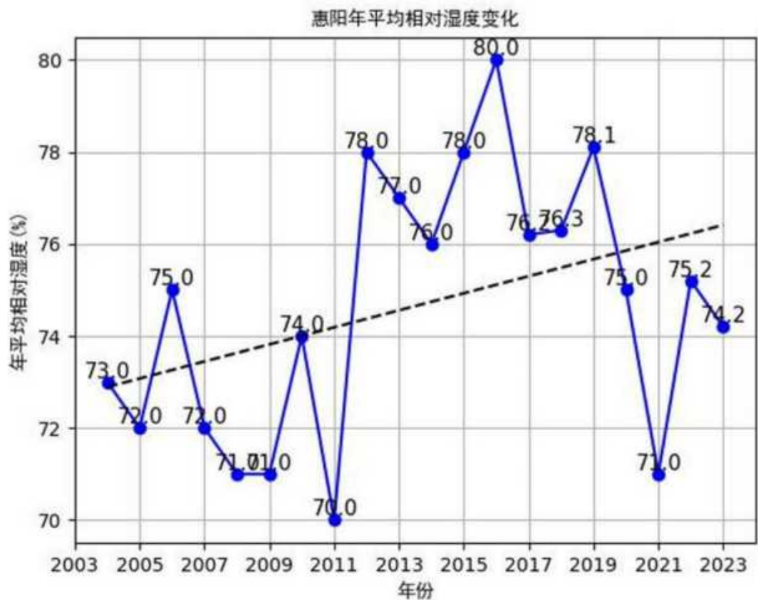
图 7.2-11 惠阳（2004-2023）年平均相对湿度（纵轴为百分比，虚线为趋势线）
