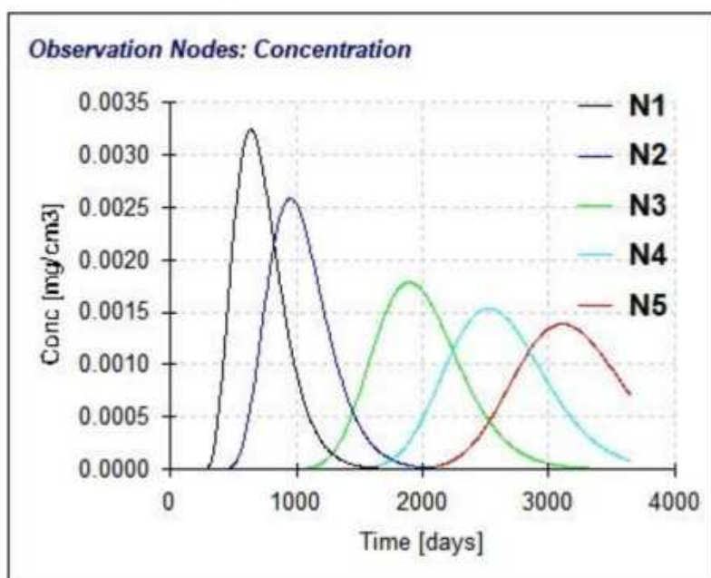
图 7.6-6 土壤不同深度石油烃浓度观测曲线
