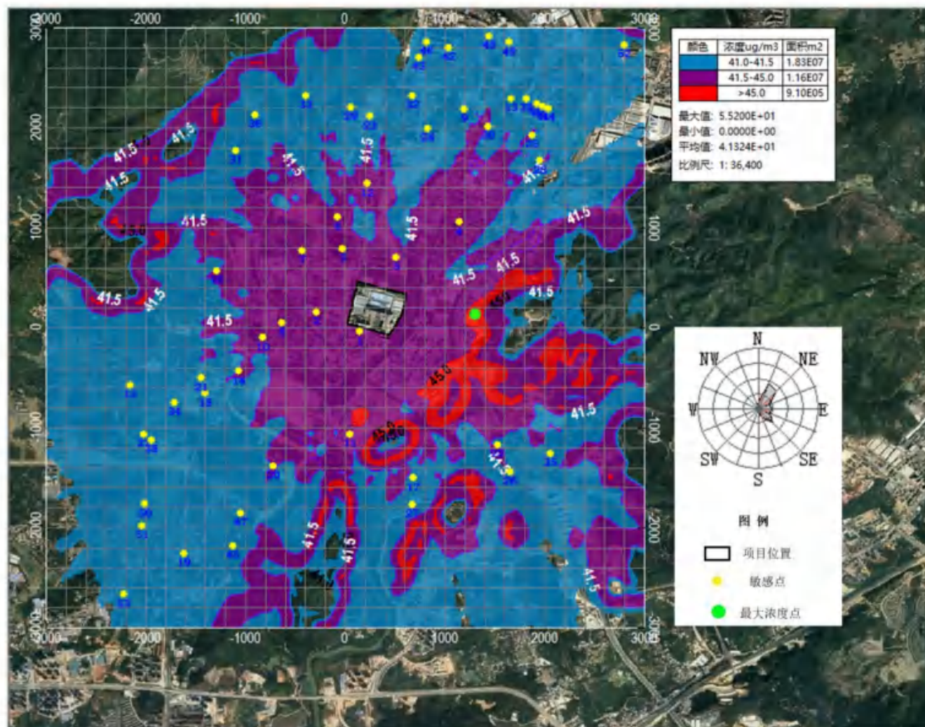
图 7.2-22 NO x 小时值平均浓度分布图
