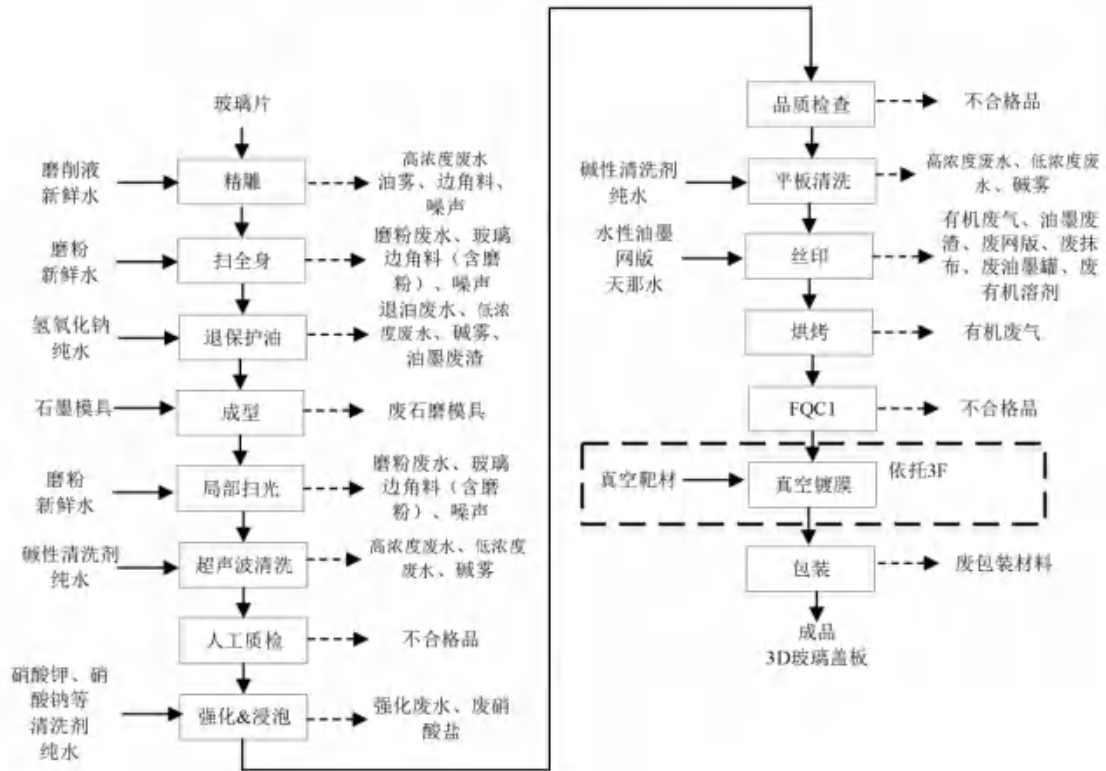
图 3.3-13 3D 玻璃盖板生产工艺流程图
