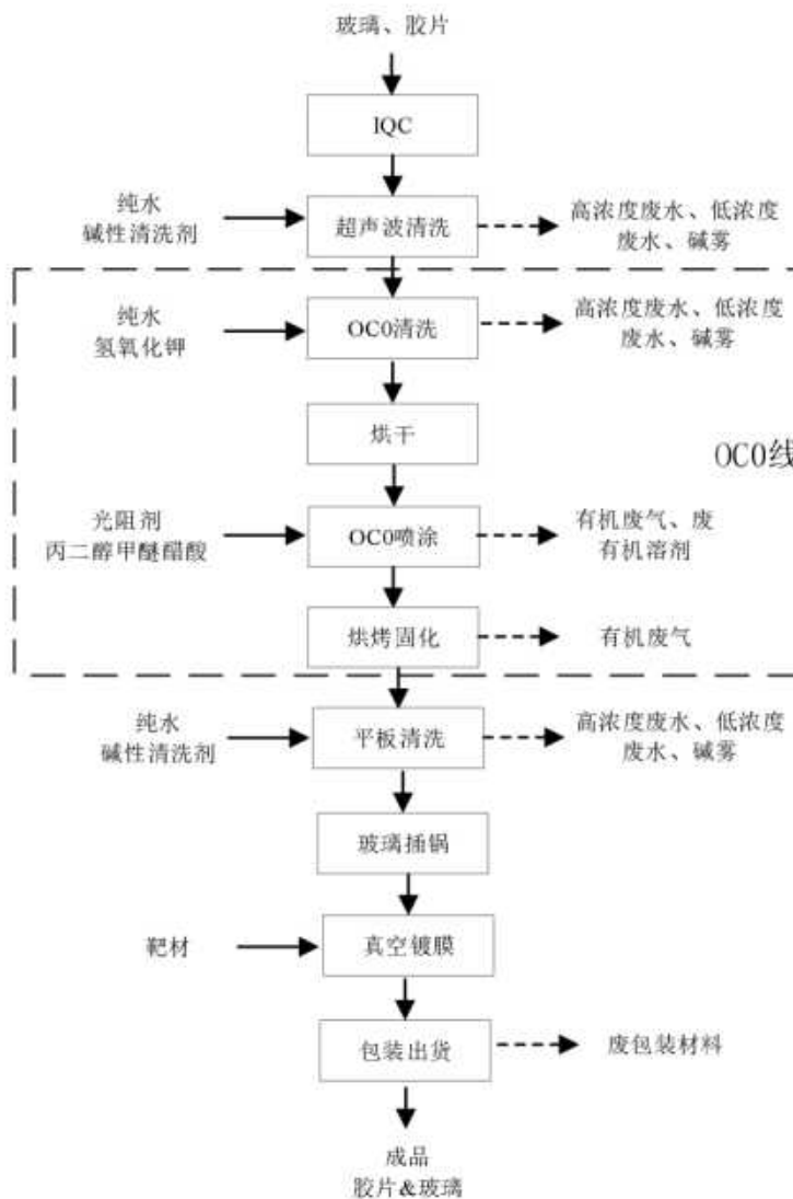
图 3.3-12 胶片&amp;玻璃加工工艺流程图
