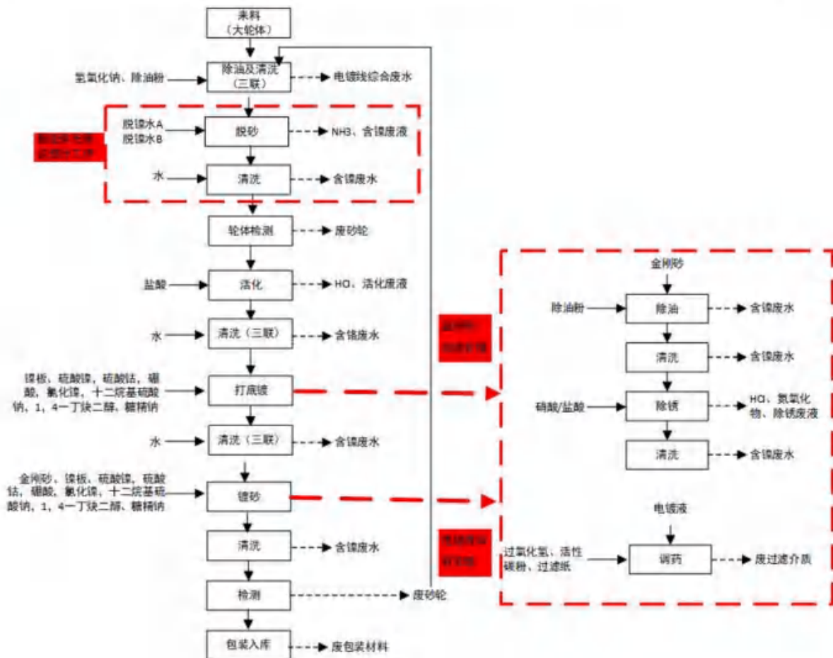
图 4.2-10 大砂轮生产工艺流程图
