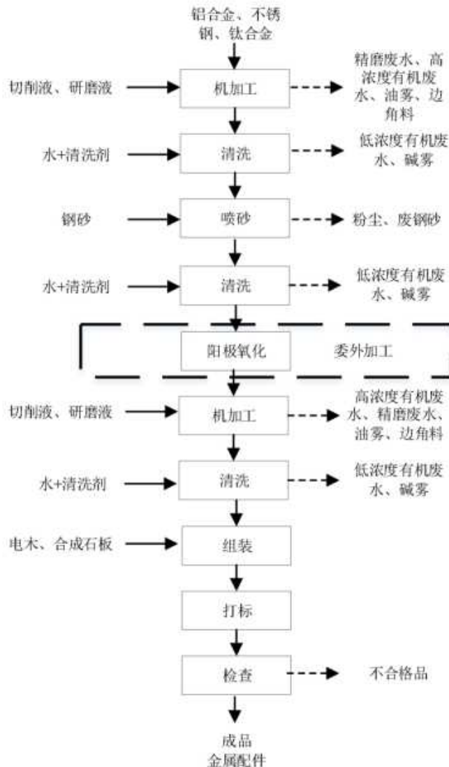
图 3.3-5 金属配件的主要生产工艺及产污节点图
