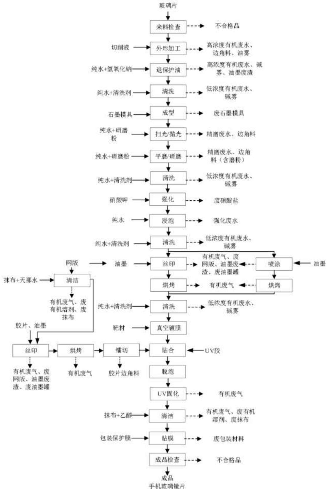
图 3.3-6 手机玻璃镜片的主要生产工艺及产污节点图 各主要工序简述：
