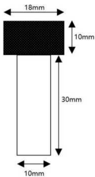
图 4.1-7 单砂轮规格尺寸图
