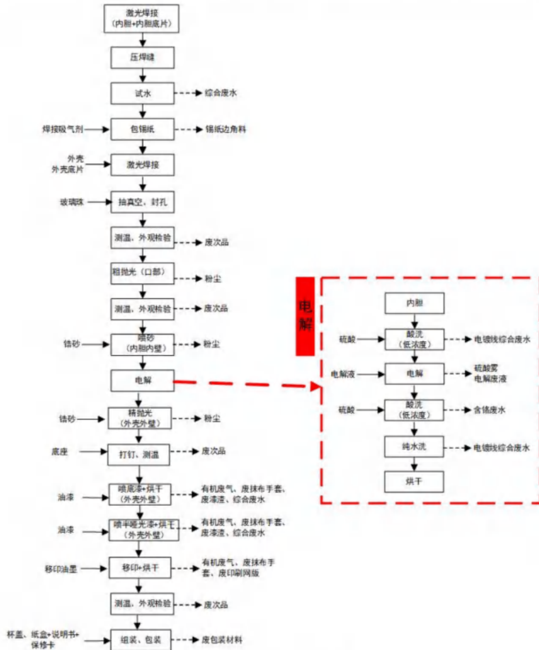
图 4.2-7 保温杯生产工艺流程图
