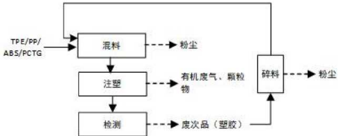
图 4.2-6 保温饭盒底座、包胶、手提盖、隔水片生产工艺流程图
