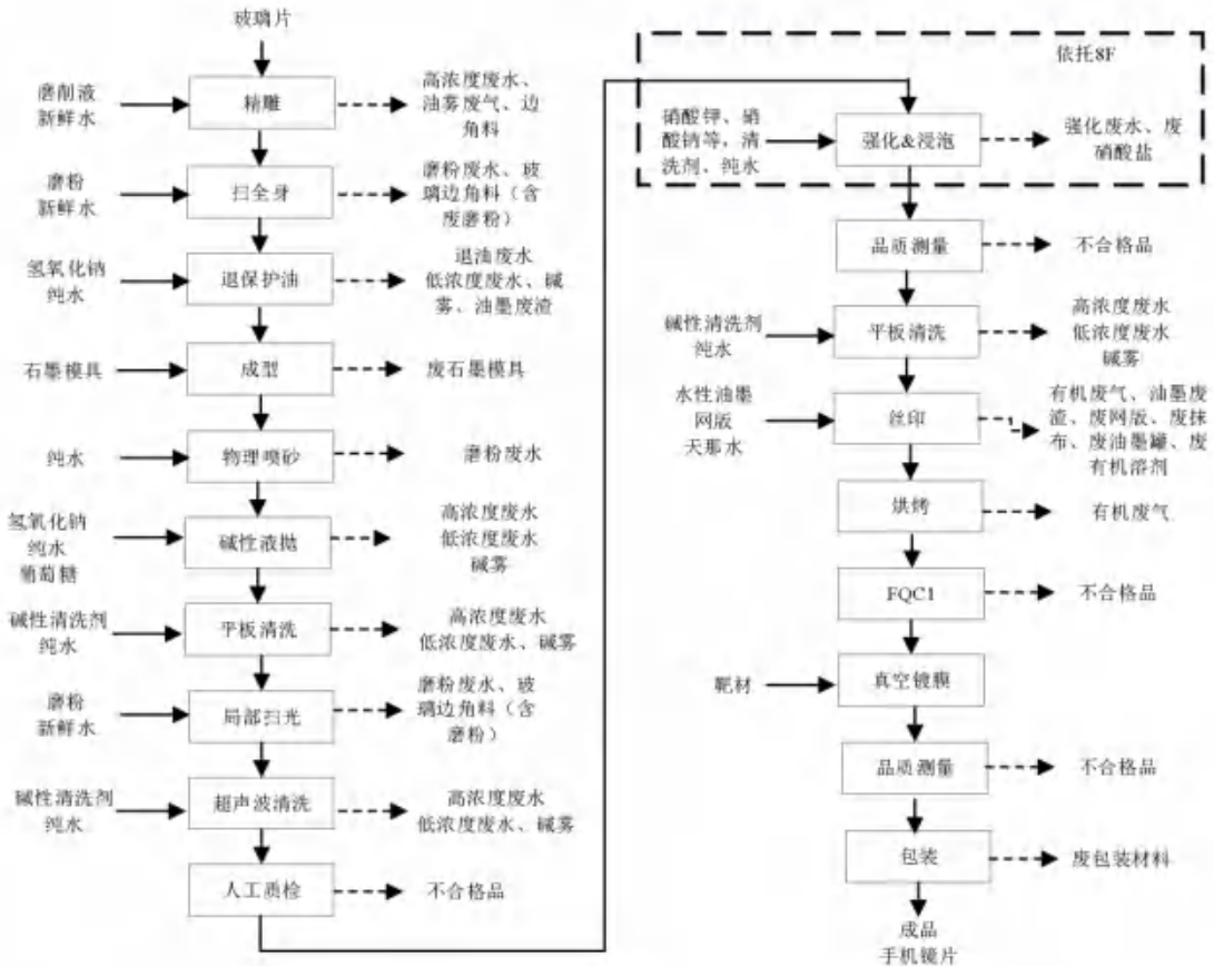
图 3.3-14 手机镜片生产工艺流程图
