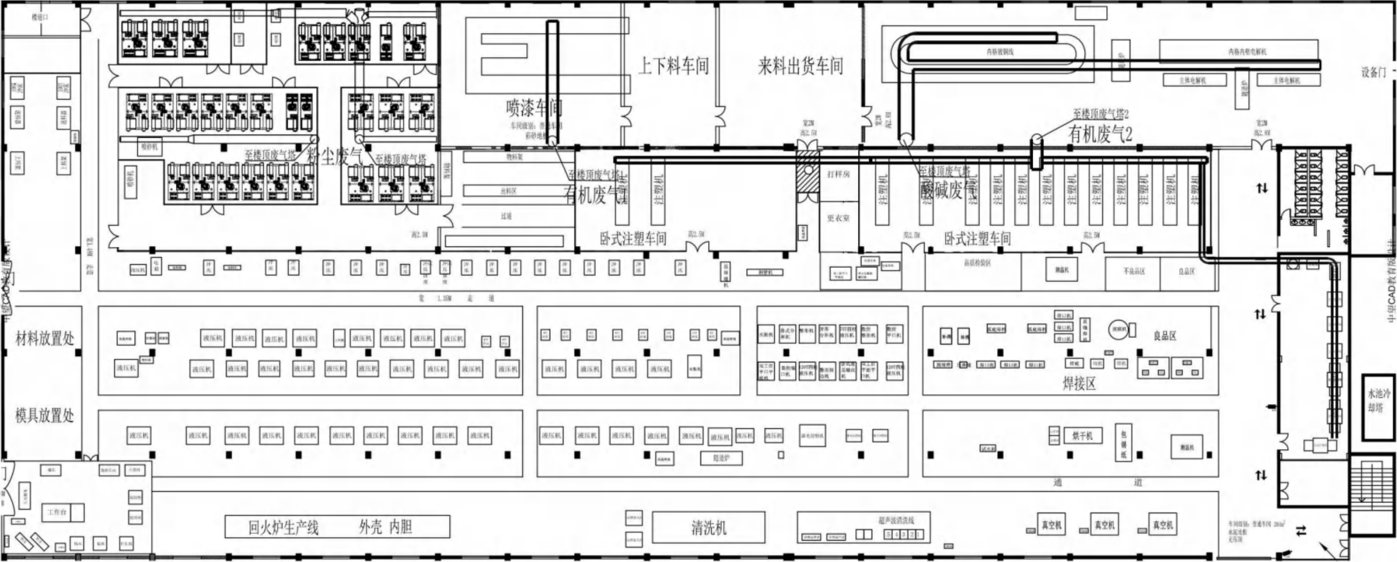
图 4.1-17 B3 厂房 1 楼车间布局图（保温杯、保温饭盒生产线）
