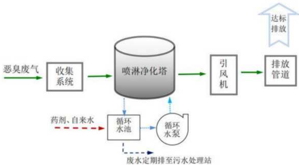
图 8.3-5 生物滤池除臭工艺流程图 a
