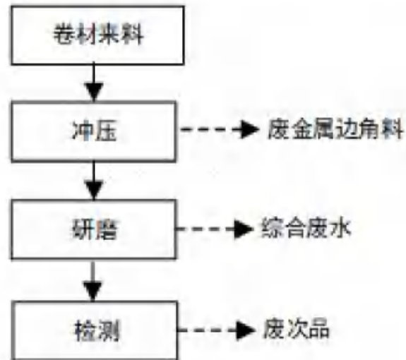
图 4.2-3 保温饭盒耳座生产工艺流程
