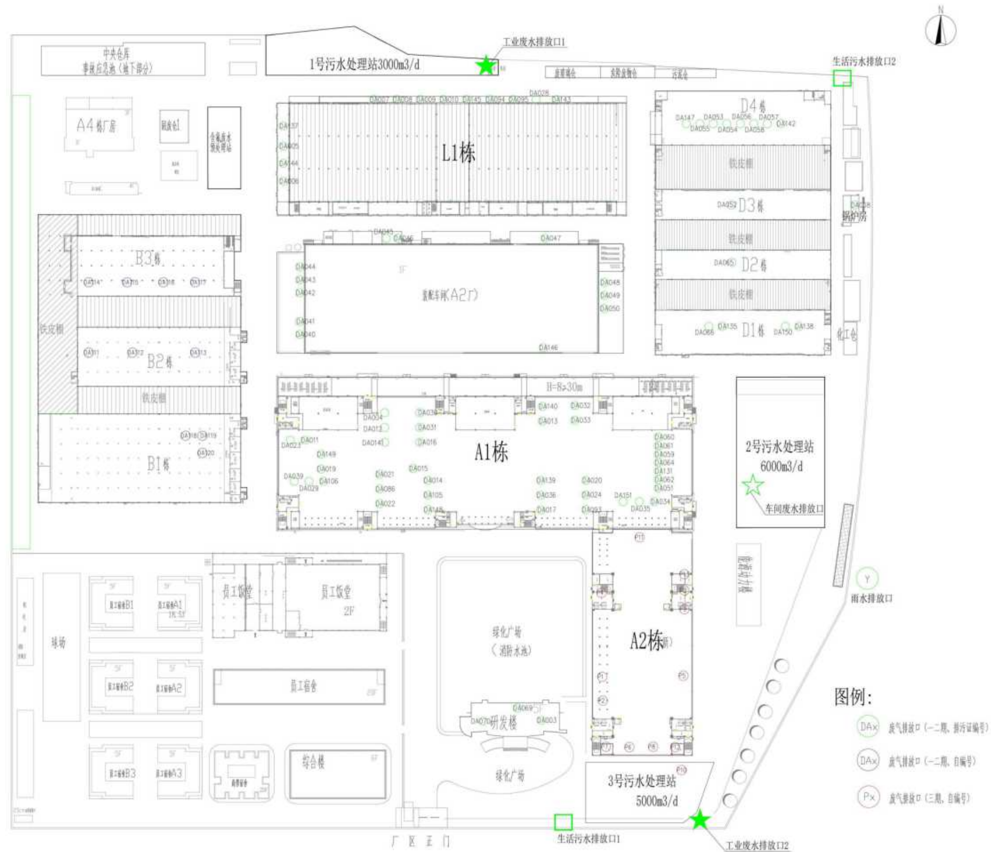
图 3.2-2 现有项目厂区平面布局图
