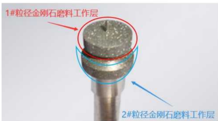
图 4.1-5 双砂轮产品图
