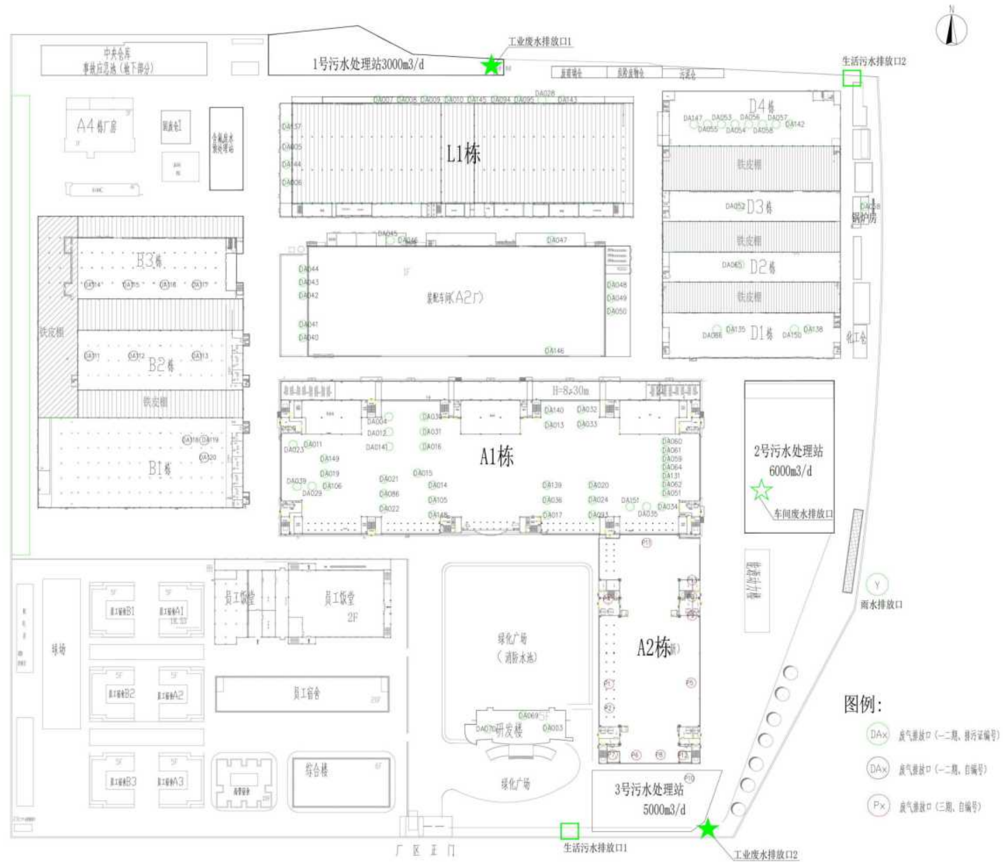
图 4.1-12 全厂总平面图
