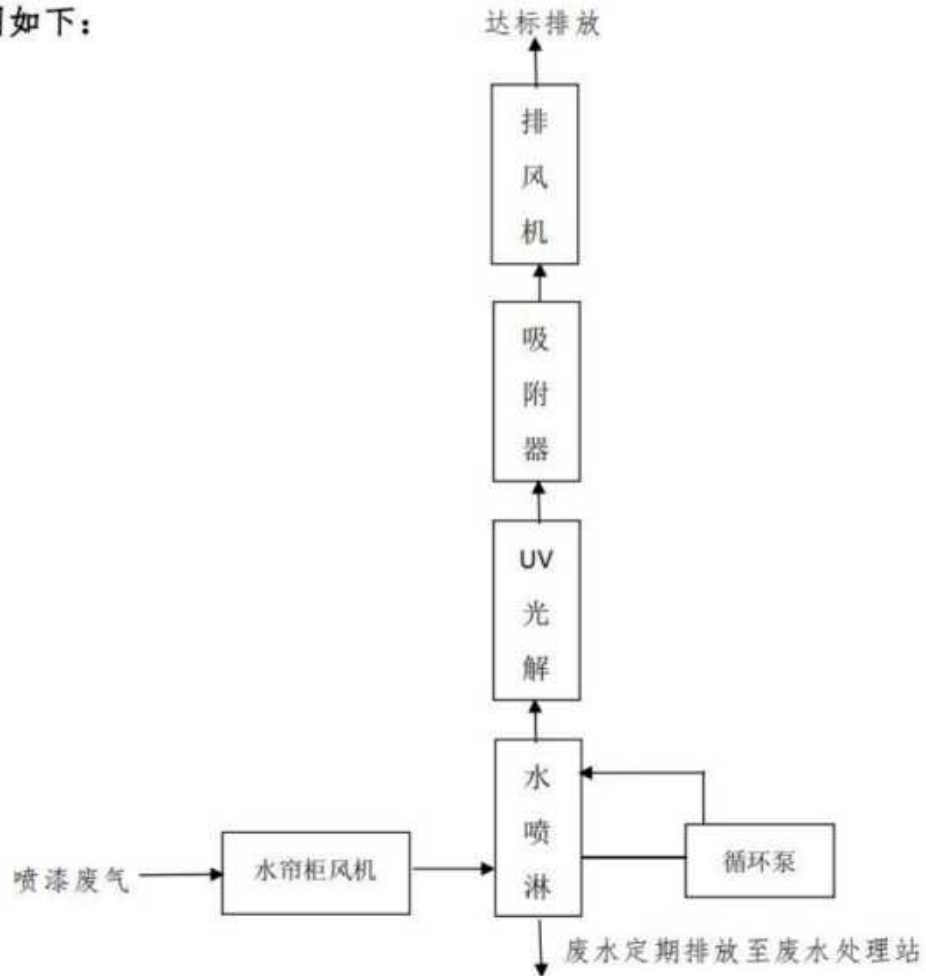
图 8.3-4 有机废气处理工艺
