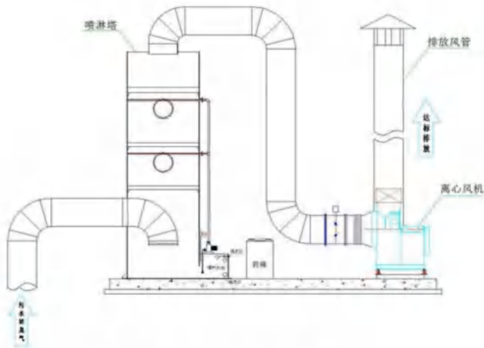
图 8.3-6 生物滤池除臭工艺流程图 a
