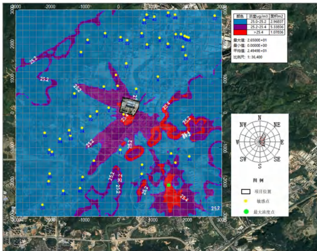
图 7.2-36 氯化氢小时值平均浓度分布图
