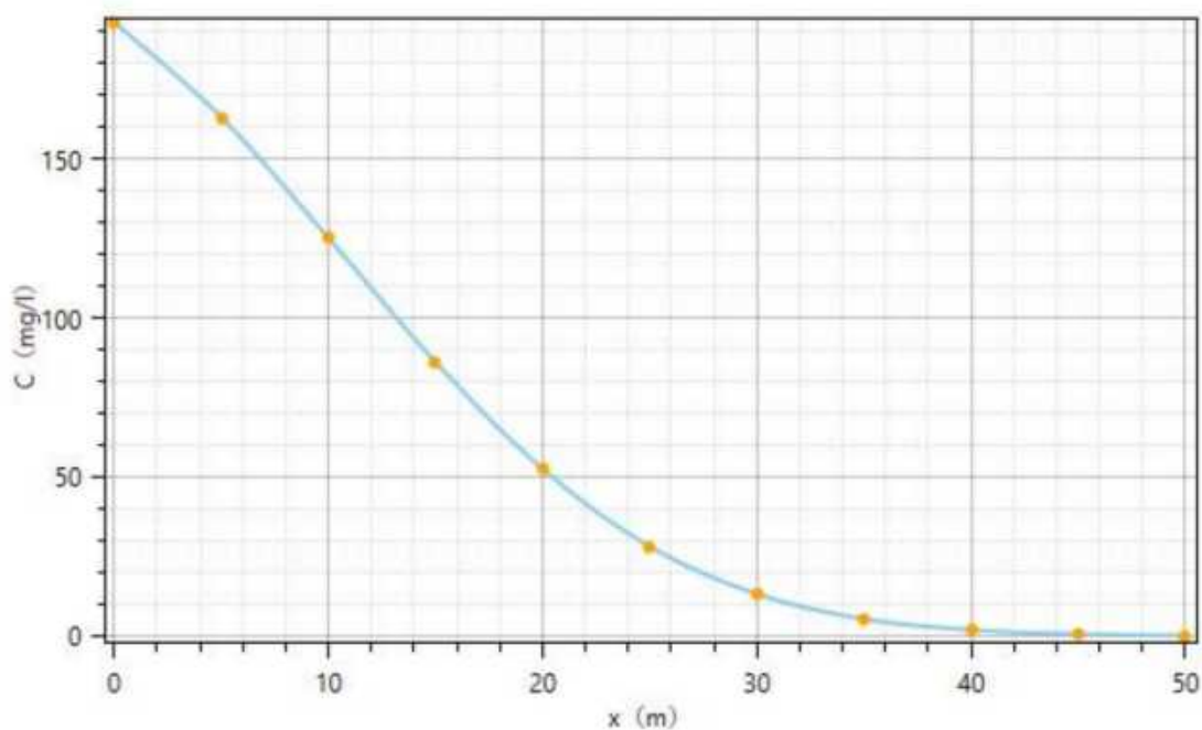
图 7.5-5 污染物镍进入含水层 365d 后情况预测统计图
