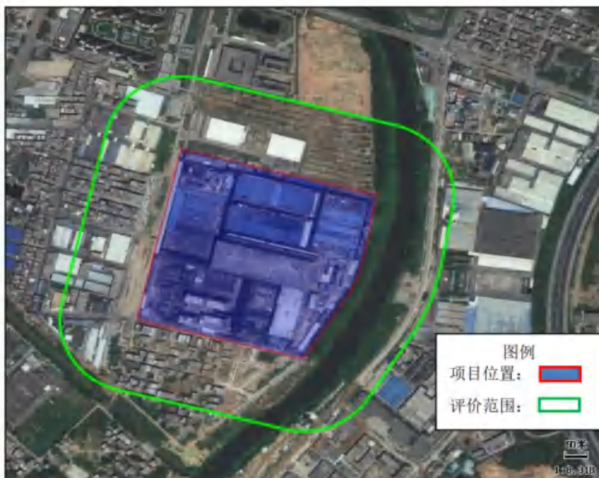
图 2.4-5 声环境评价范围
