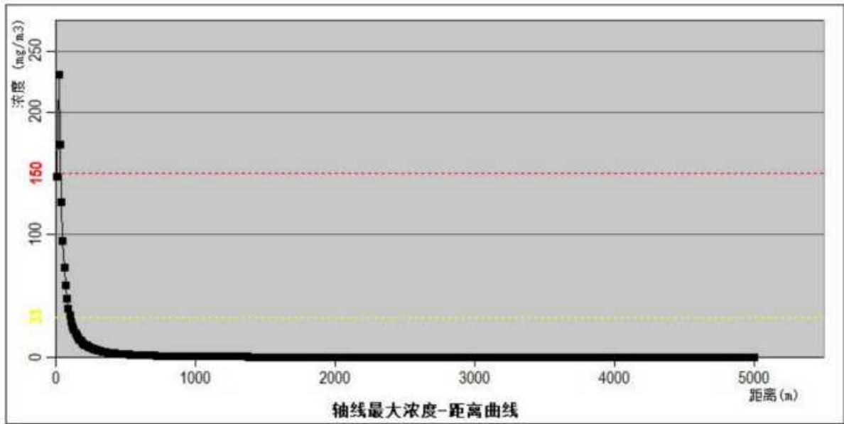
图 9.6-1 氯化氢泄漏事故排放在下风向不同距离处的最大浓度（最不利气象条件）
