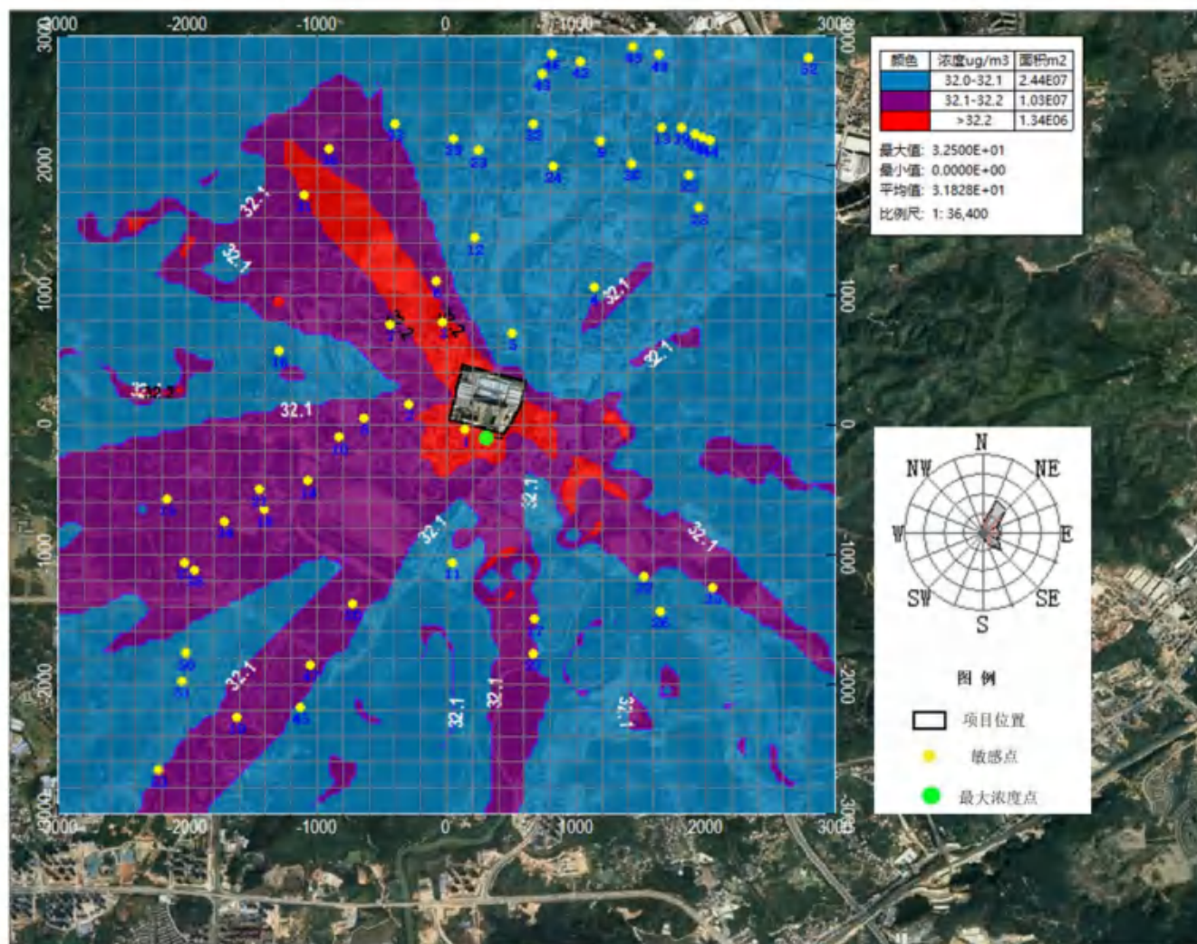
图 7.2-20 NO 2 日平均浓度分布图
