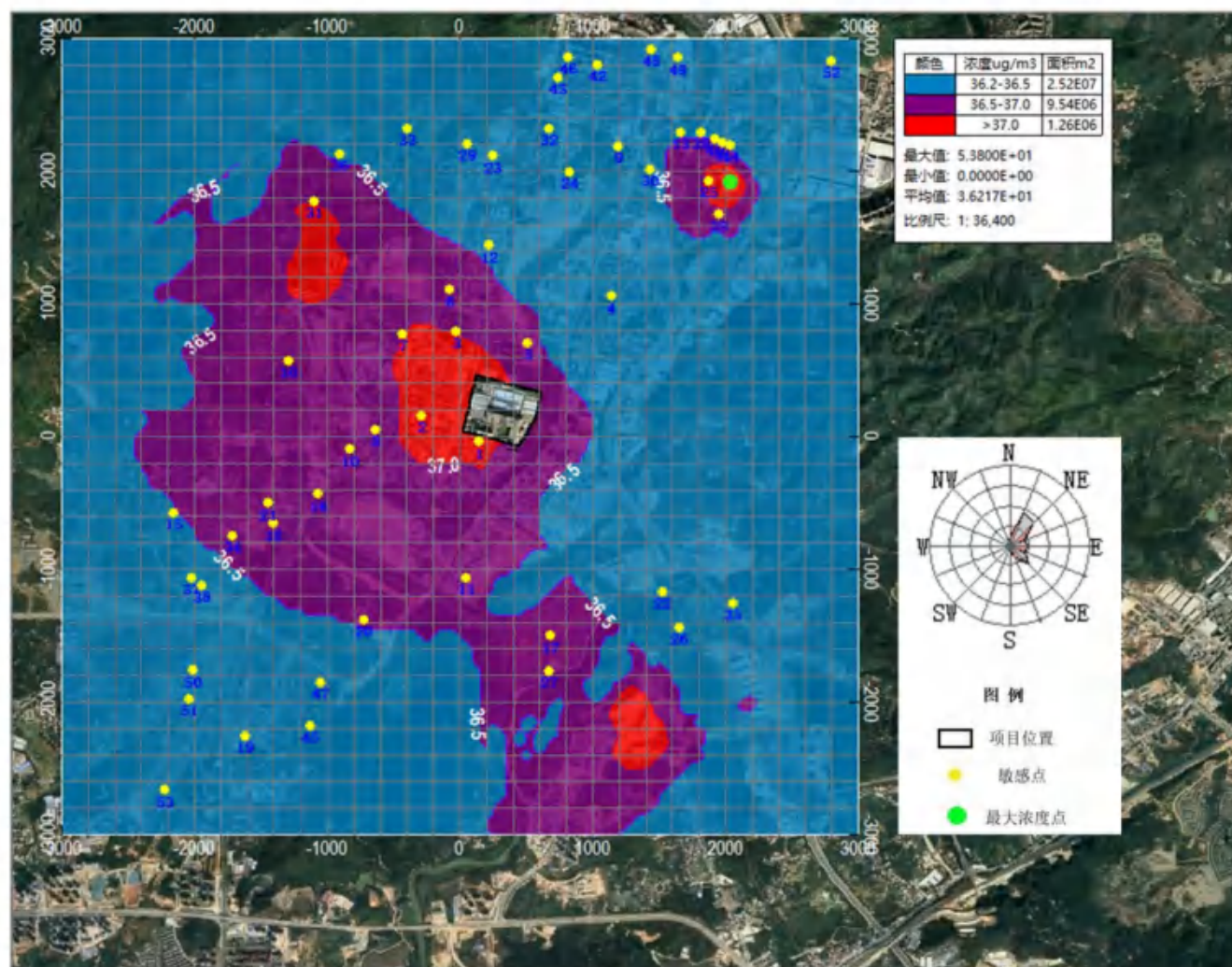
图 7.2-28 PM10 年平均浓度分布图
