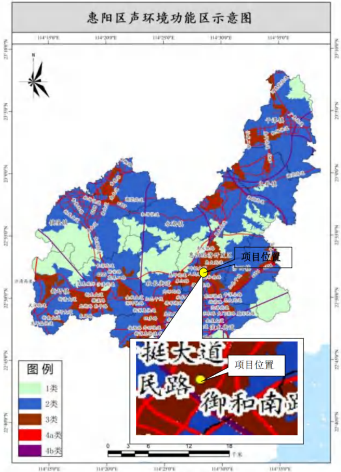
图 2.3-3 声环境质量功能区划图
