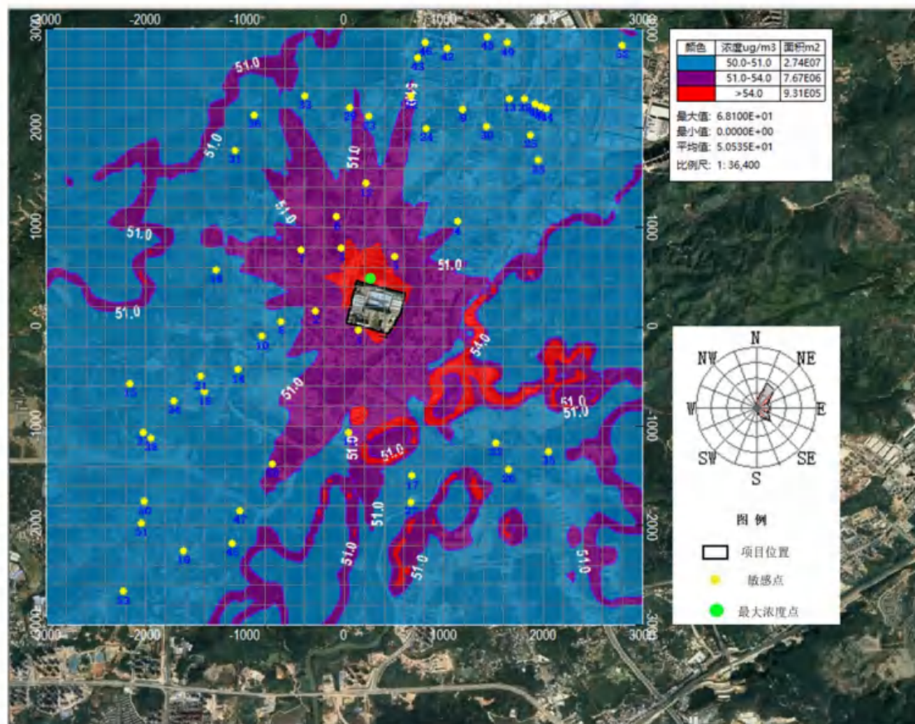
图 7.2-33 NH 3 小时值平均浓度分布图
