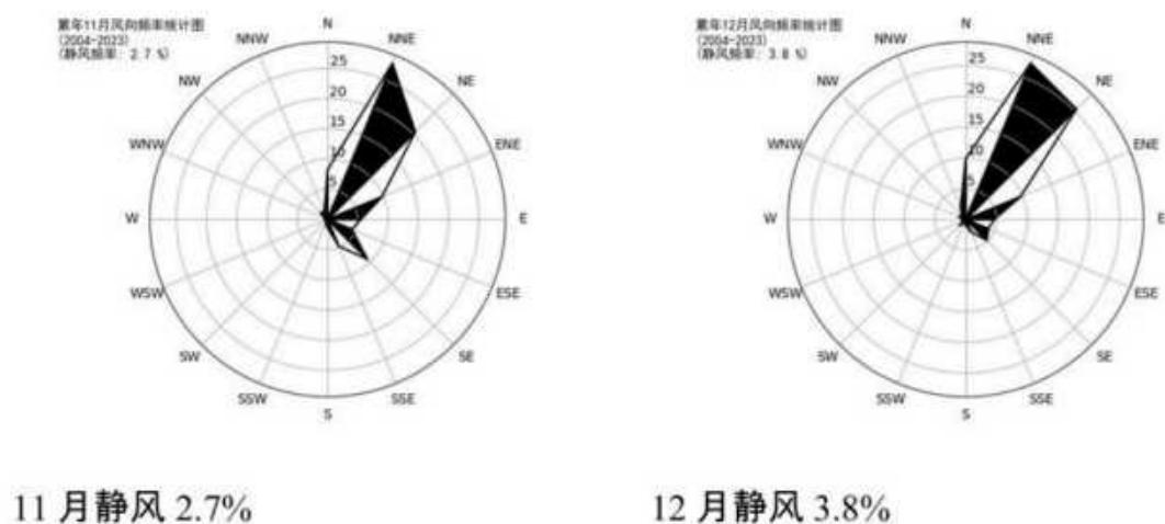
图 7.2-2 惠阳站月风向玫瑰图
