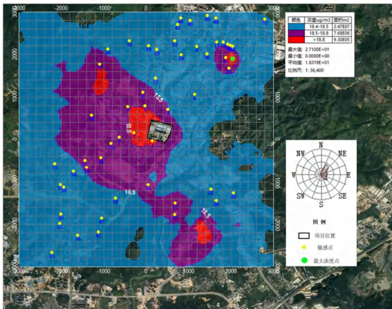
图 7.2-30 PM2.5 年平均浓度分布图
