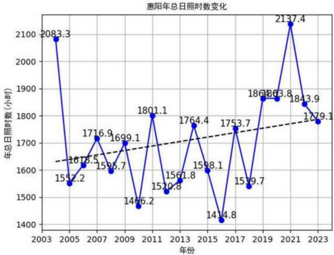
图 7.2-9 惠阳（2004-2023）年日照时长（单位：小时，虚线为趋势线）
