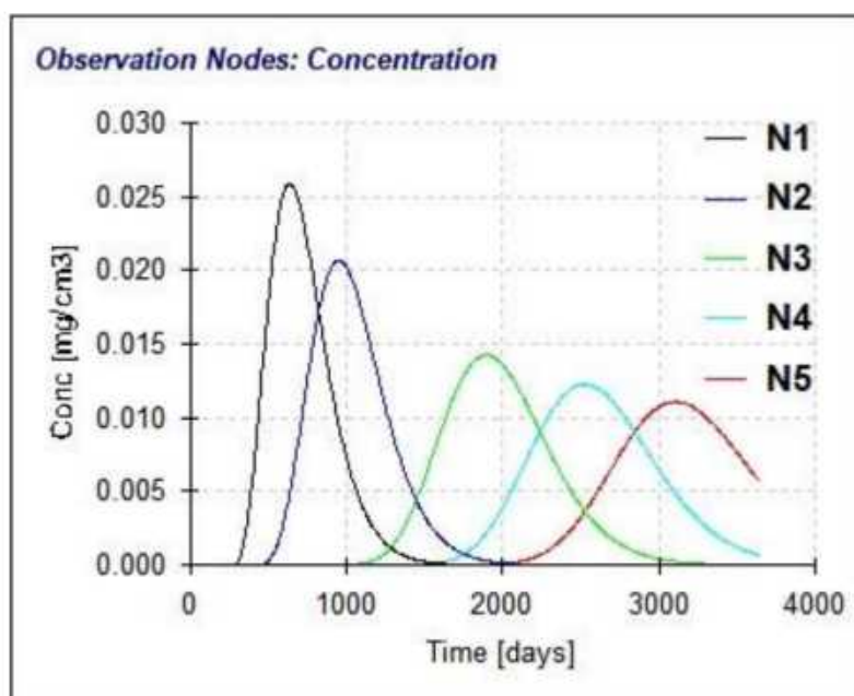
图 7.6-2 土壤不同深度铜离子浓度观测曲线
