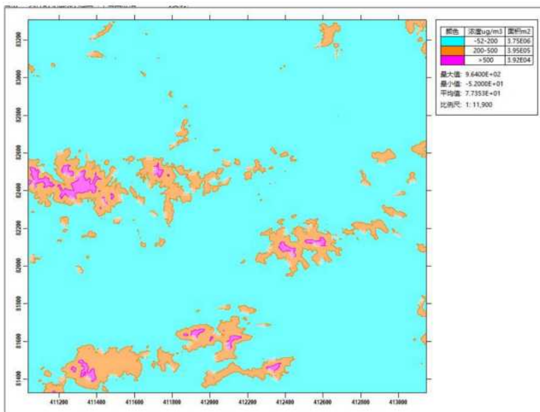
图 2.4-3 地形数据的取值范围内的地形示意图（高程单位：m、面积单位：m 2 ）
