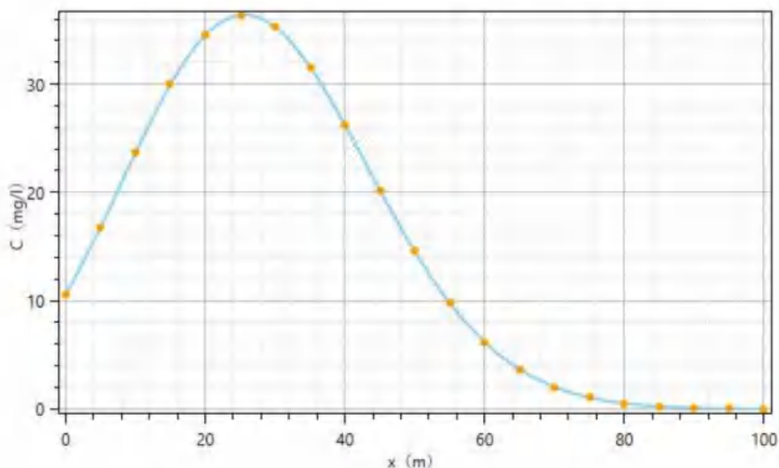
图 7.5-6 污染物镍进入含水层 1000d 后情况预测统计图
