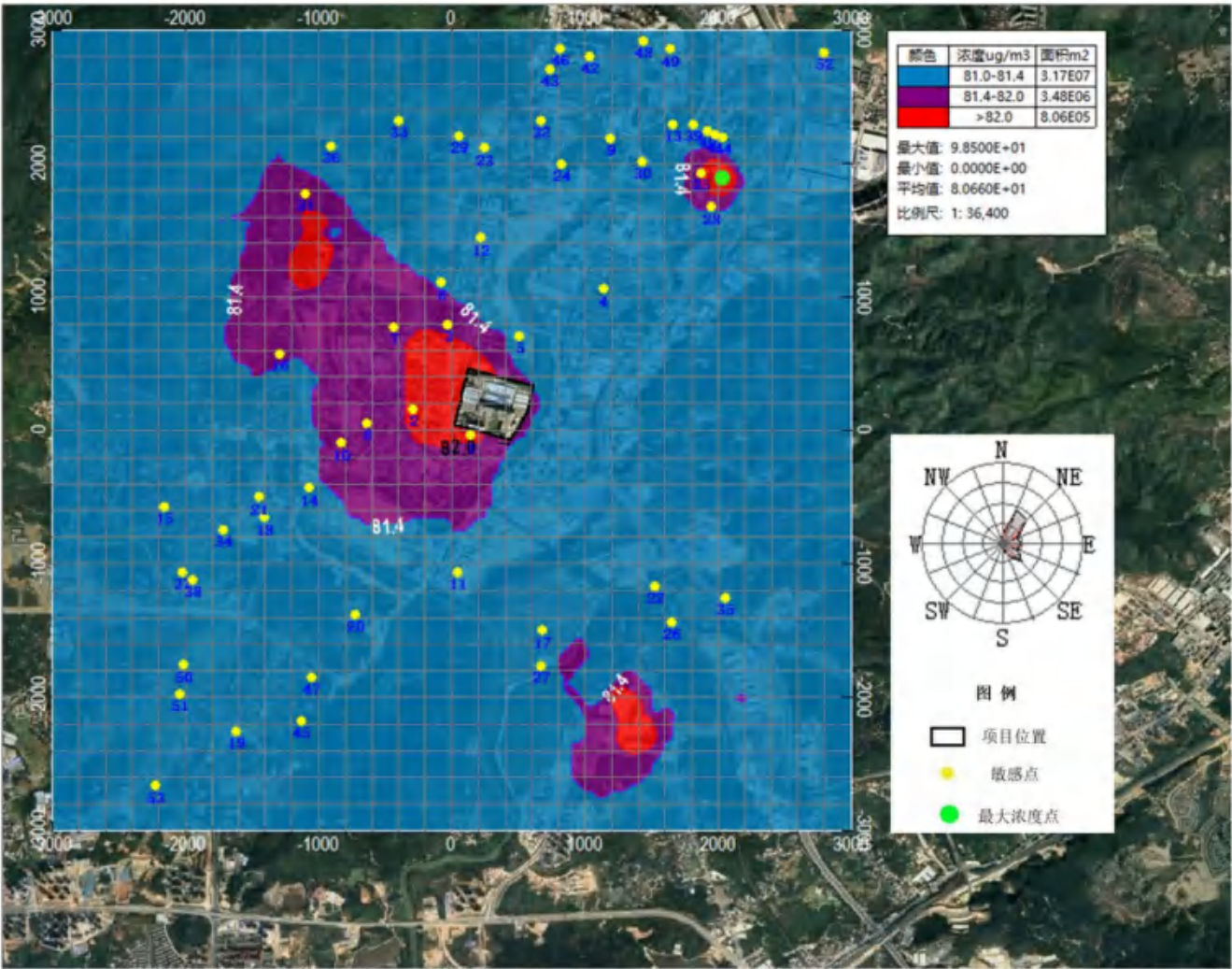
图 7.2-26 TSP 年平均浓度分布图
