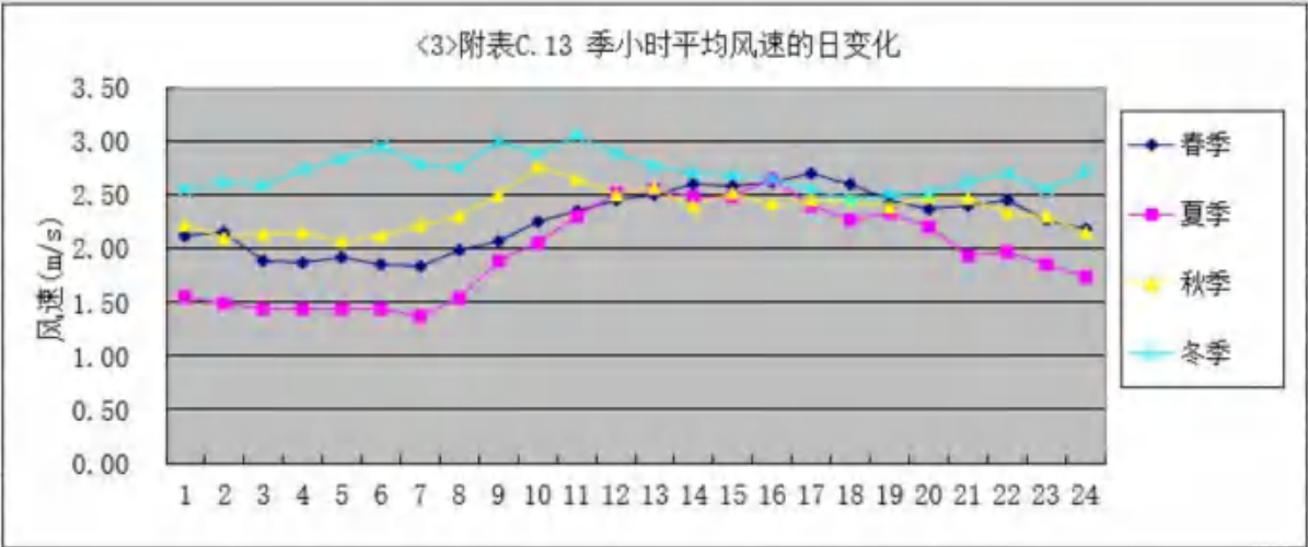
图 7.2-14 惠阳气象站季小时平均风速的日变化图
