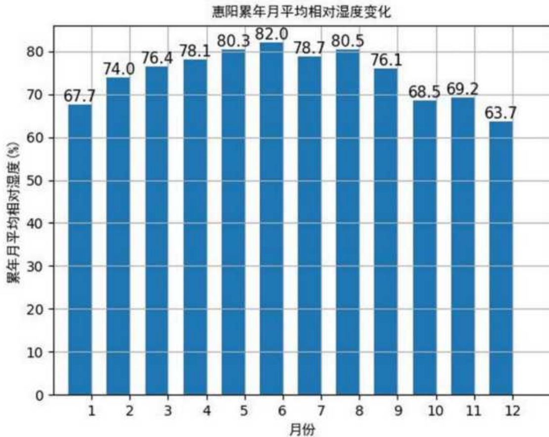
图 7.2-10 惠阳月平均相对湿度（纵轴为百分比）
