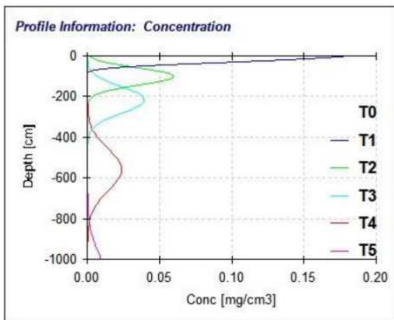
图 7.6-5 镍离子在不同水平天沿土壤迁移曲线
