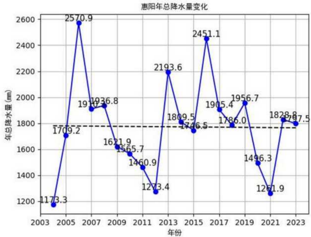
图 7.2-7 惠阳（2004-2023）年总降水量（单位：毫米，虚线为趋势线）
