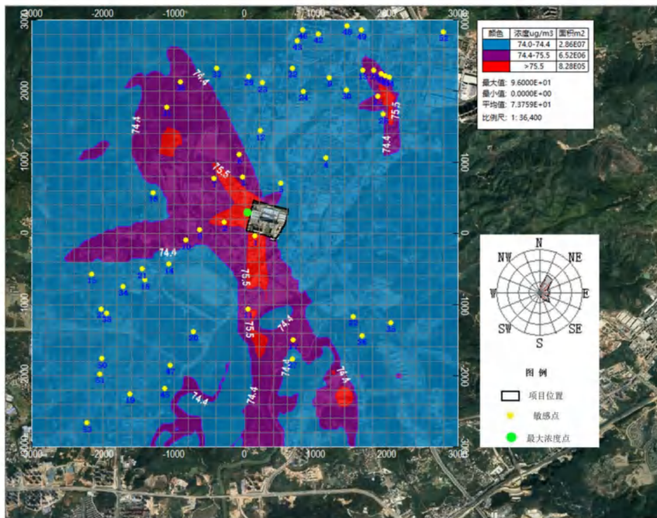
图 7.2-27 PM10 日平均浓度分布图
