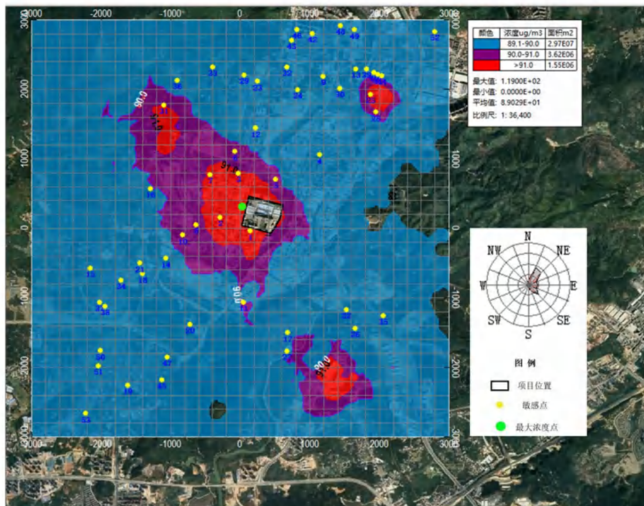
图 7.2-25 TSP 日平均浓度分布图
