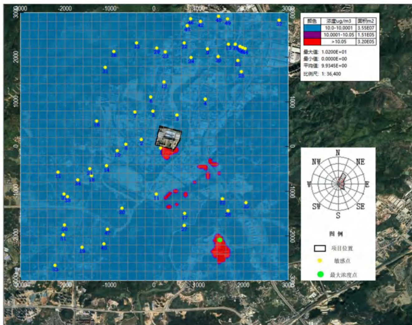
图 7.2-37 氟化氢日平均浓度分布图
