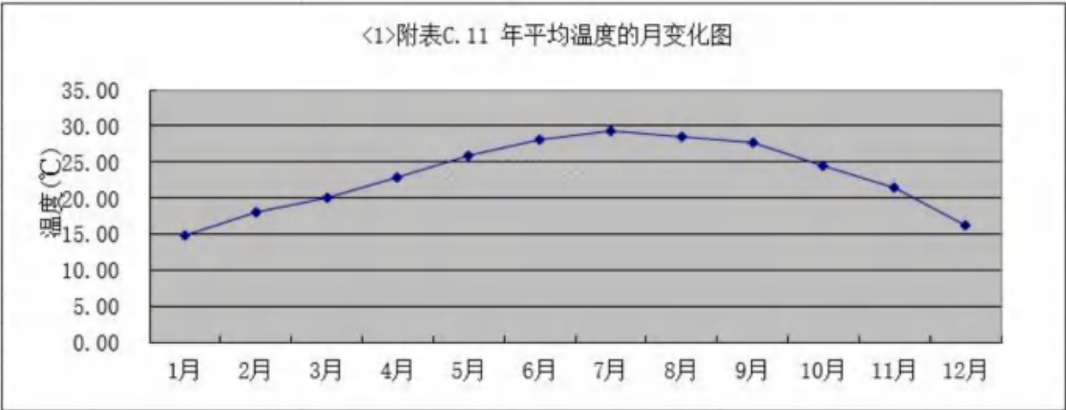
图 7.2-12 惠阳气象站年平均温度的月变化图
