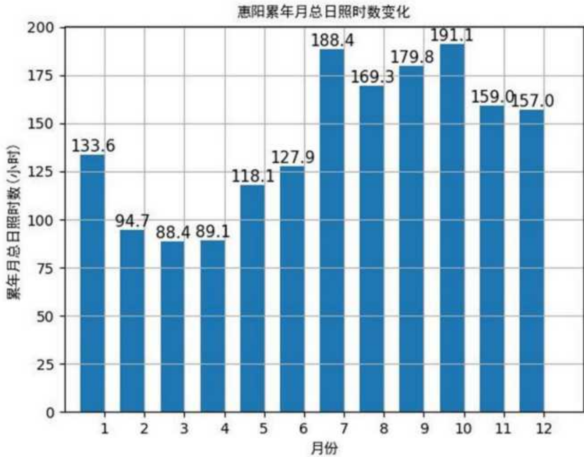
图 7.2-8 惠阳月日照时数（单位：小时）
