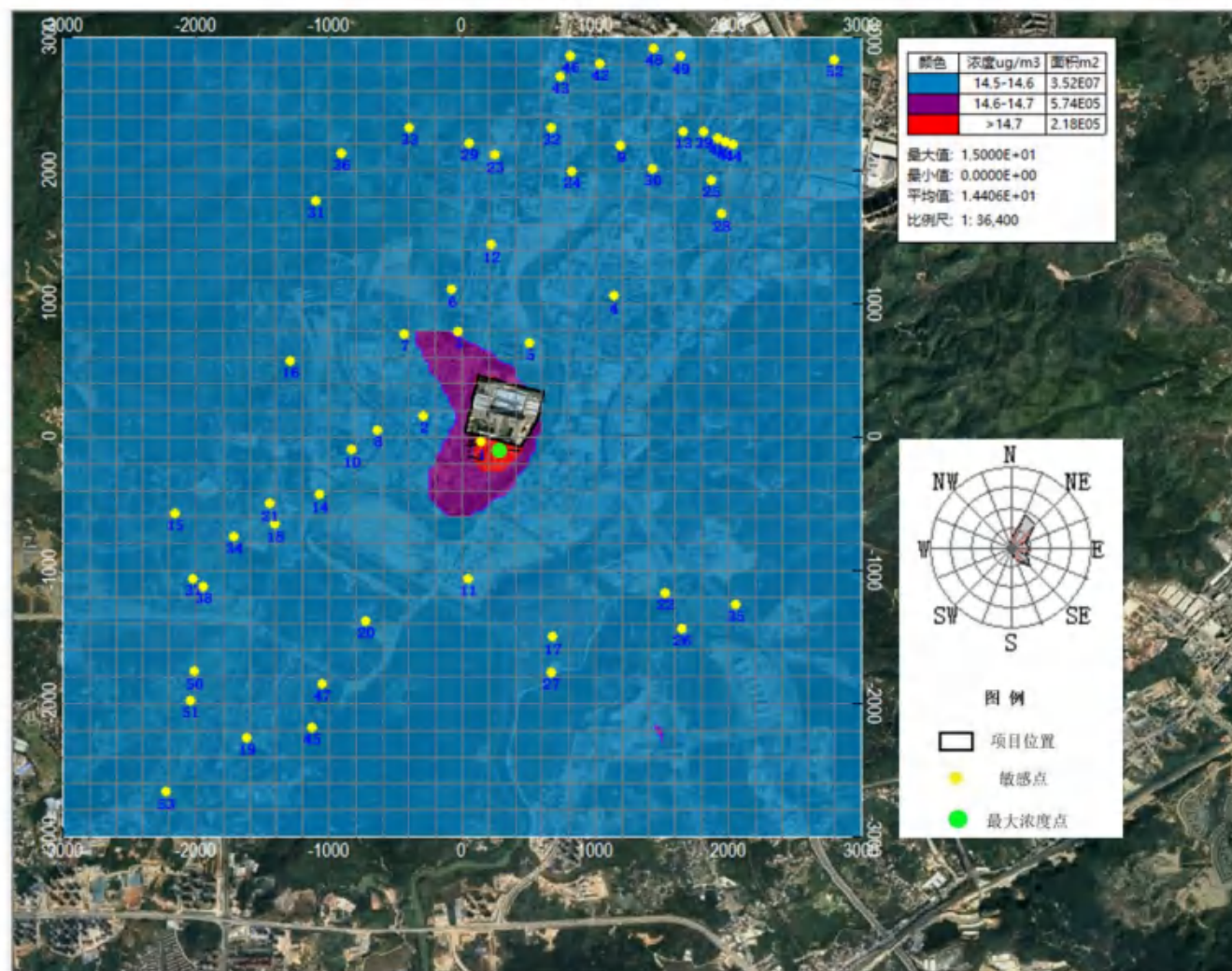
图 7.2-21 NO 2 年平均浓度分布图
