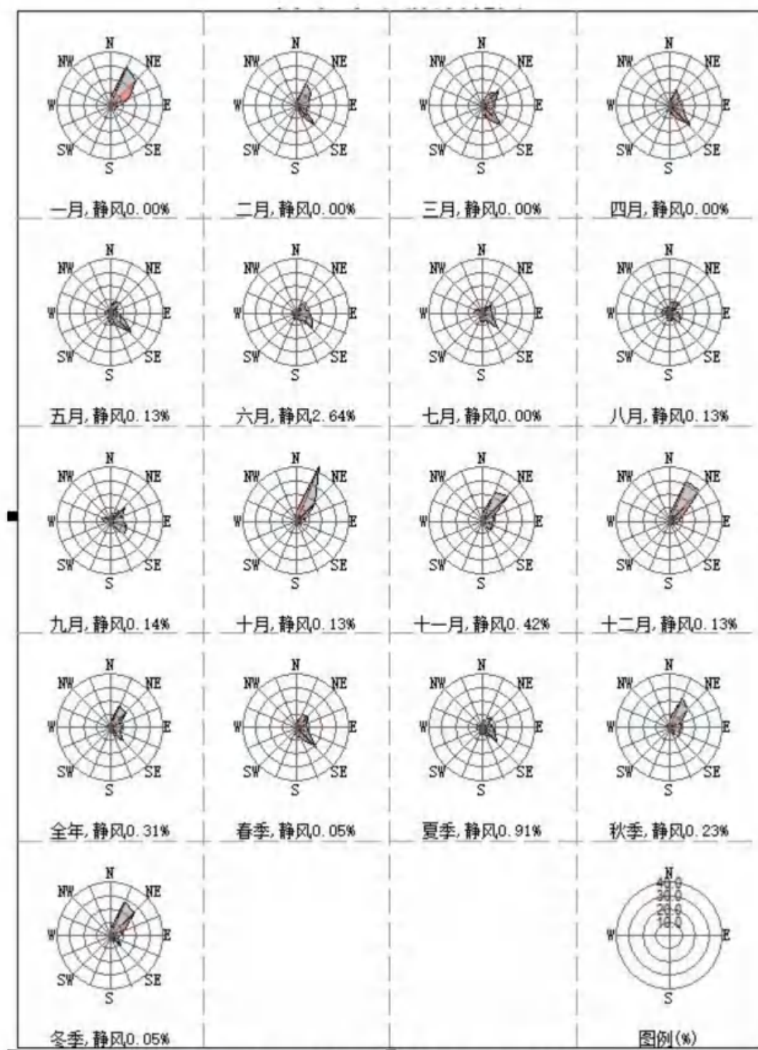
图 7.2-15 惠阳 2023 年各季及年平均风向玫瑰图
