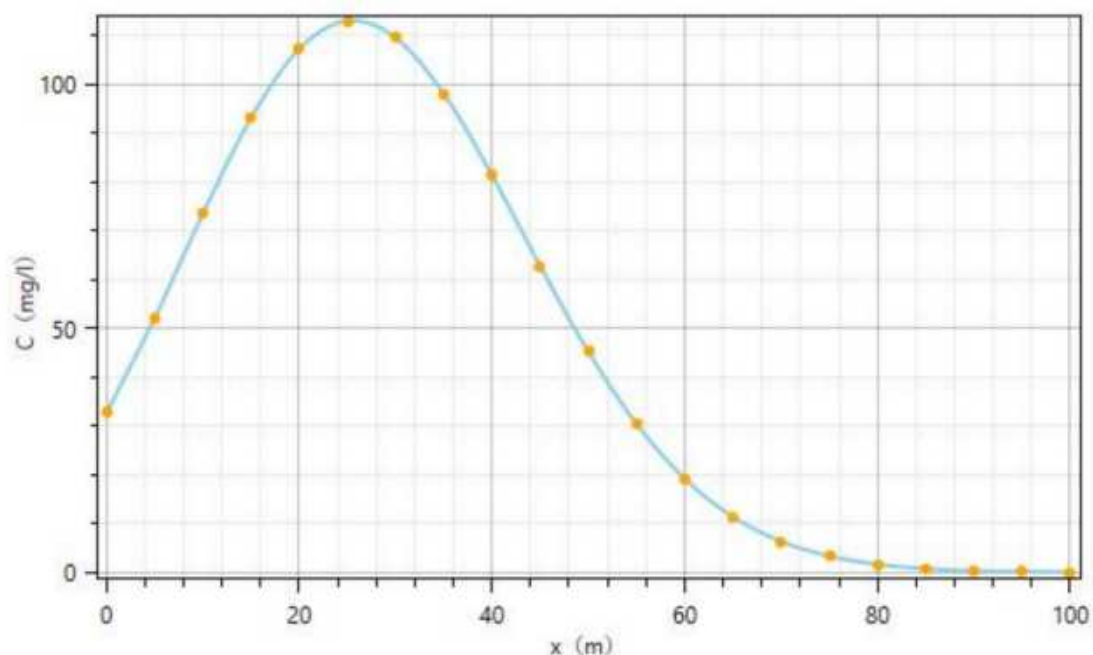
图 7.5-2 污染物 \text{COD}_{\text{Cr}} 进入含水层 1000d 后情况预测统计图
