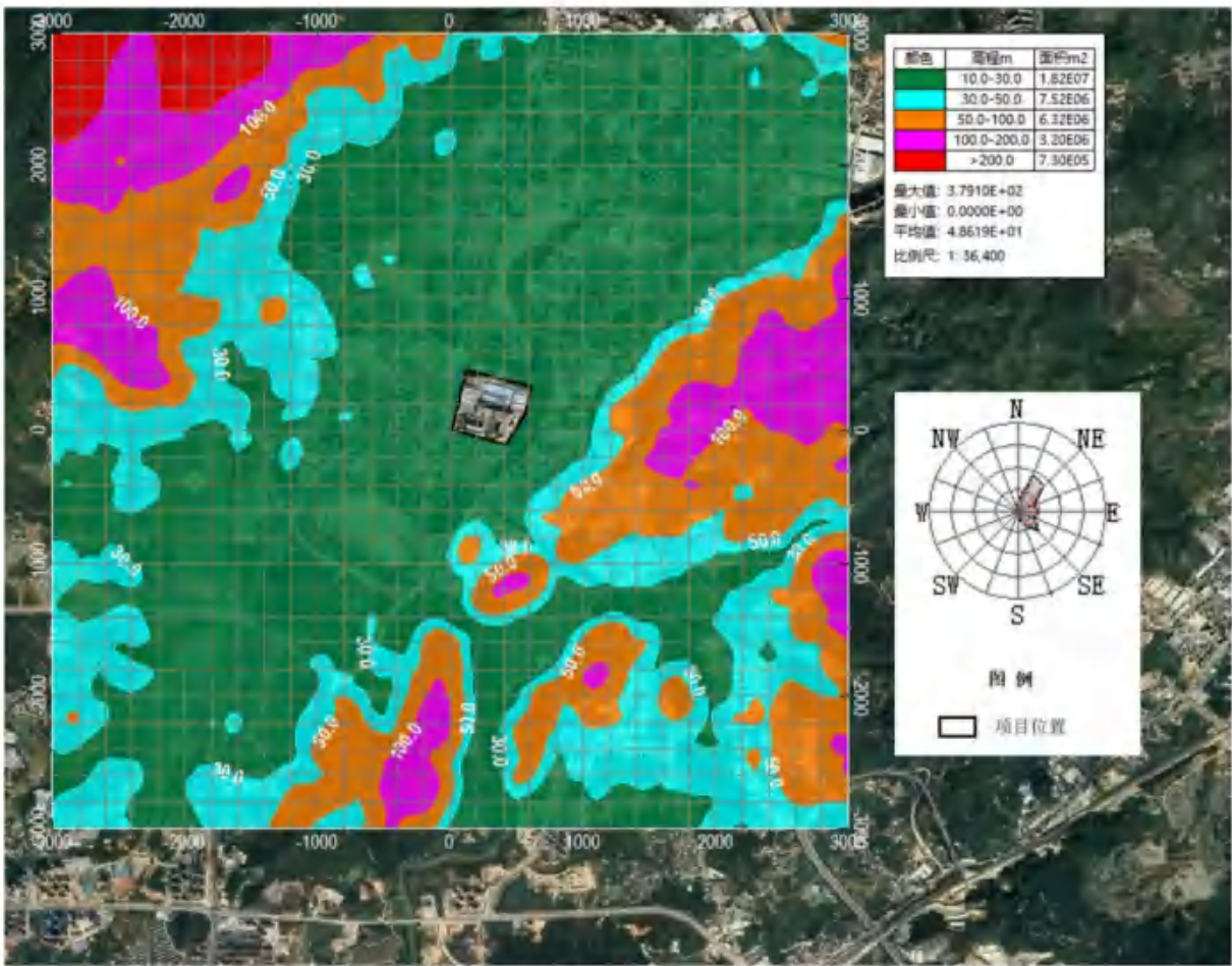
图 7.2-16 评价范围内的地形示意图（高程单位：m、面积单位：m2）
