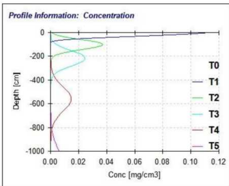
图 7.6-3 铜离子在不同水平天沿土壤迁移曲线
