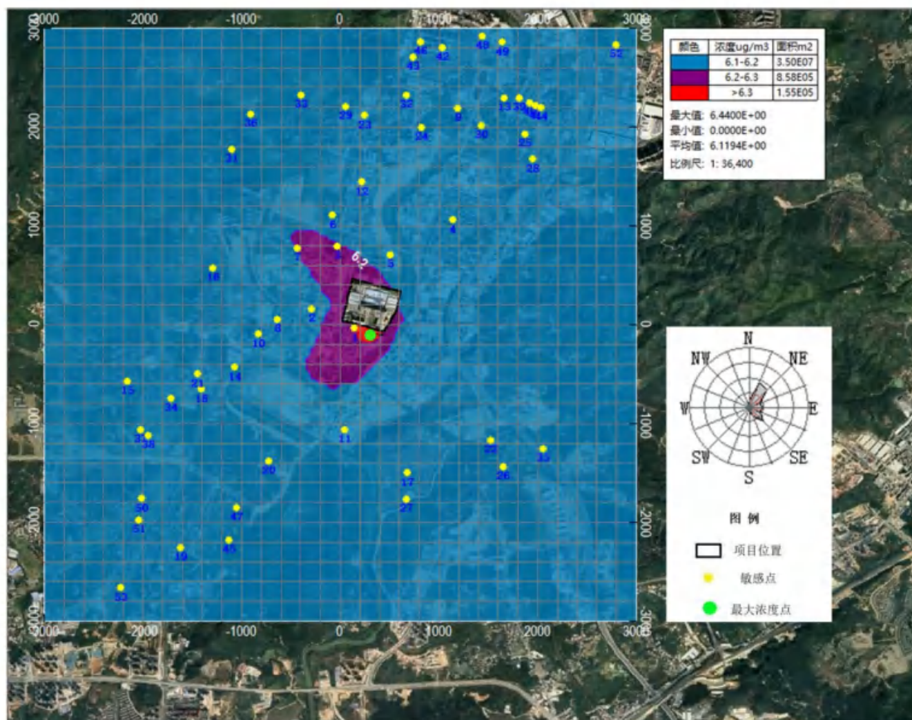
图 7.2-19 SO 2 年平均浓度分布图
