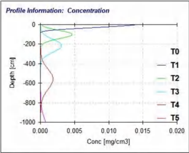
图 7.6-7 石油烃在不同水平天沿土壤迁移曲线
