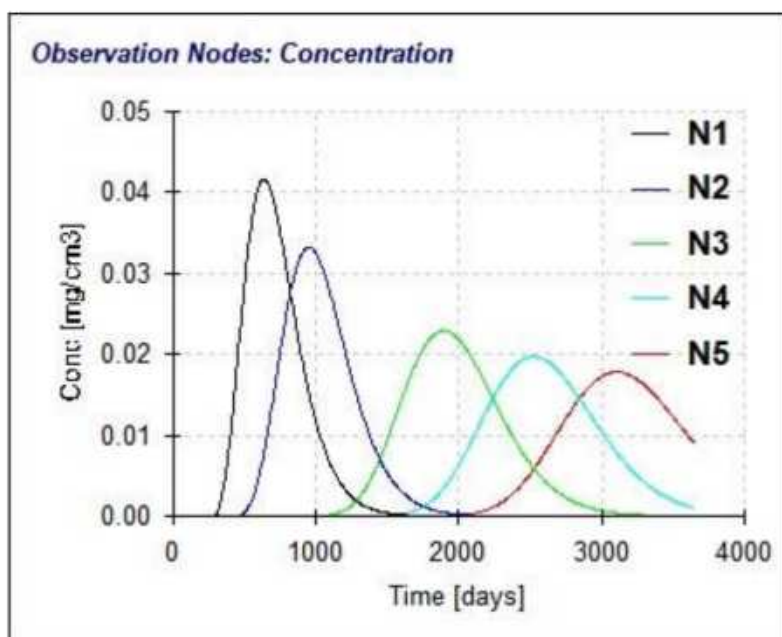
图 7.6-4 土壤不同深度镍离子浓度观测曲线
