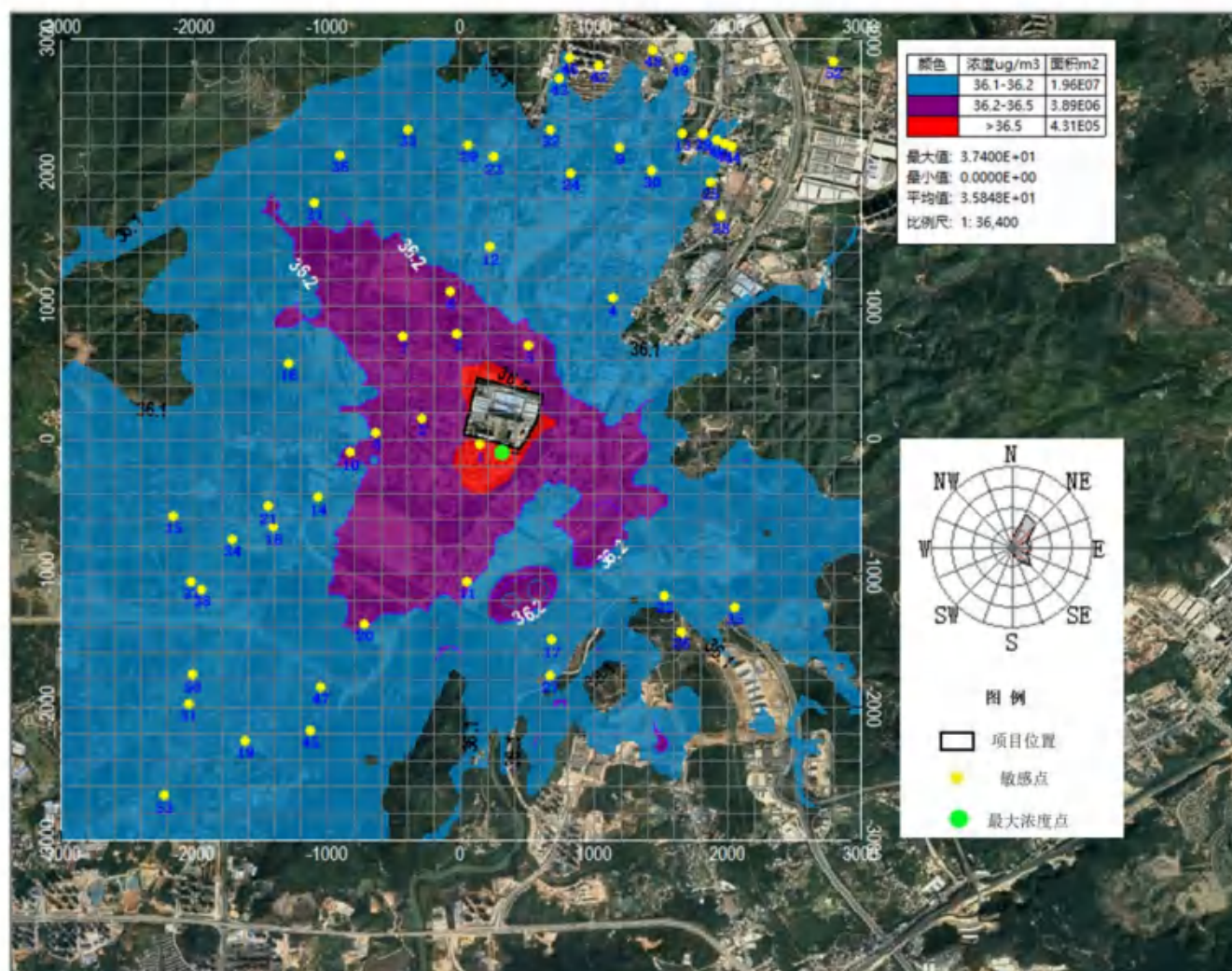
图 7.2-23 NO x 日平均浓度分布图
