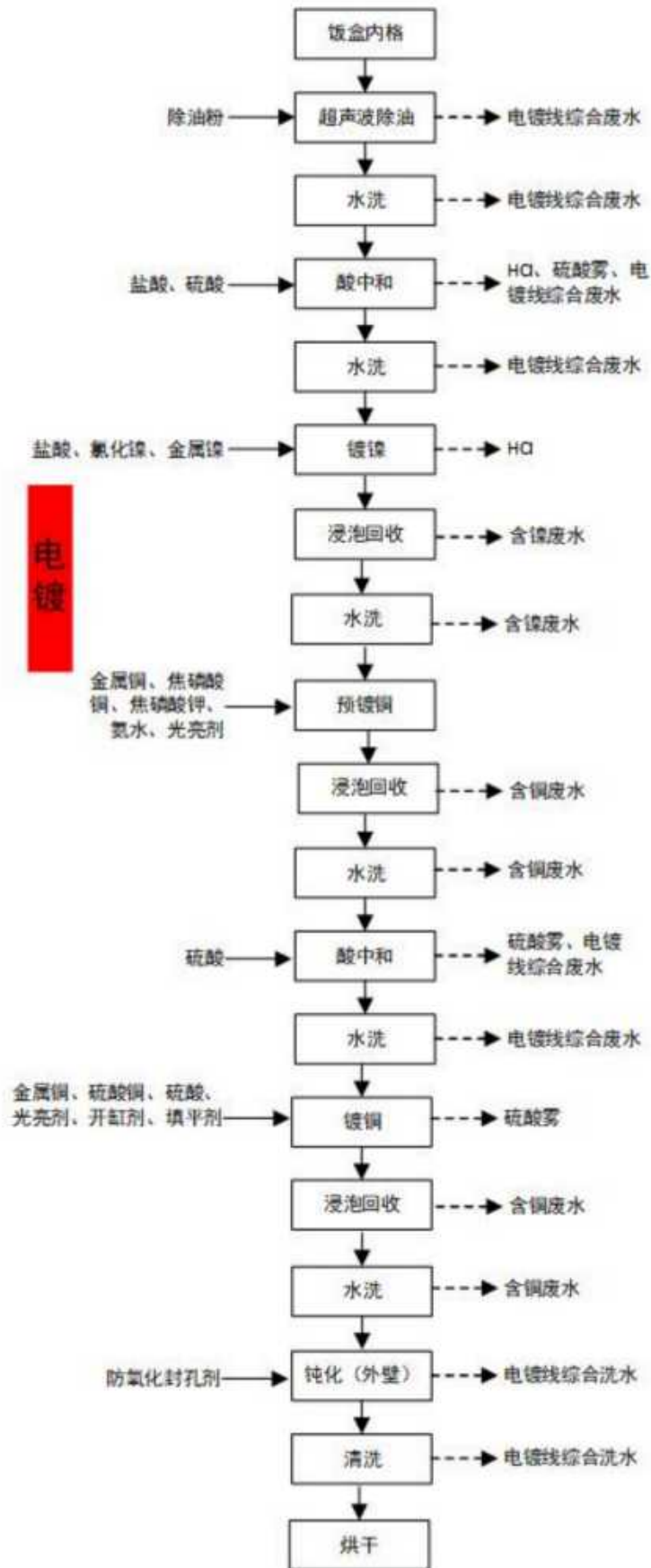
图 4.2-5 保温饭盒内格电镀工艺流程图
